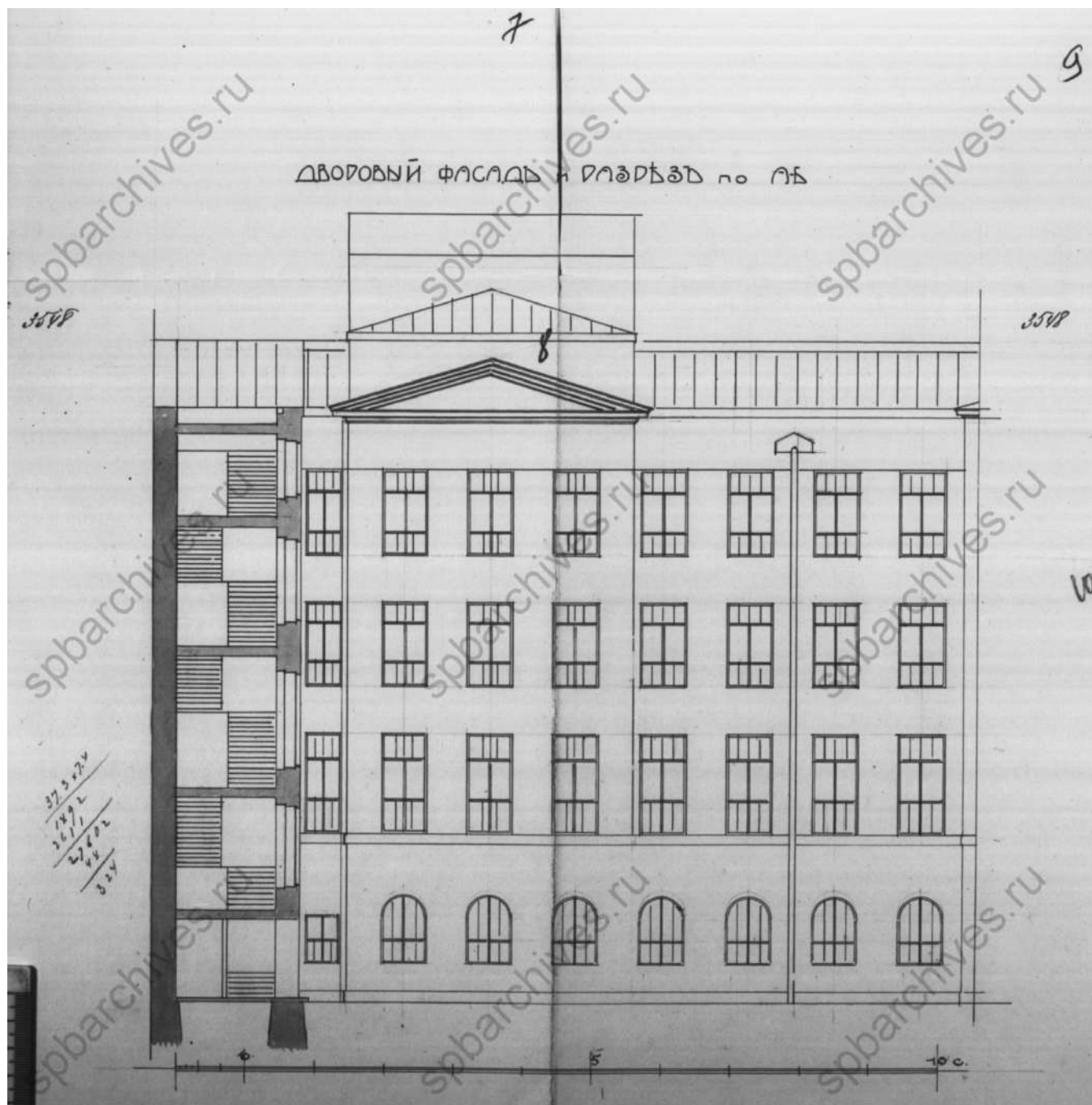
76. Дворовой фасад и разрез по АБ. 1912 г. // Источник: ЦГИА СПб Ф.515 Оп.4 Д.2911 Лл.7-10.
