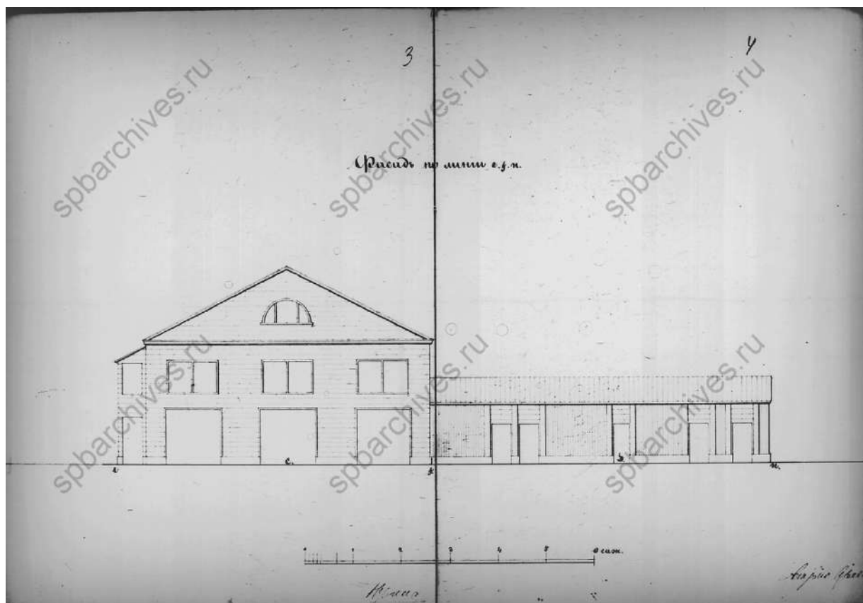
5. Фасад по линии е.п. Строения С и D. 1862 г. // Источник: ЦГИА СПб Ф.513 Оп.102 Д.1870 Лл.3, 4.
