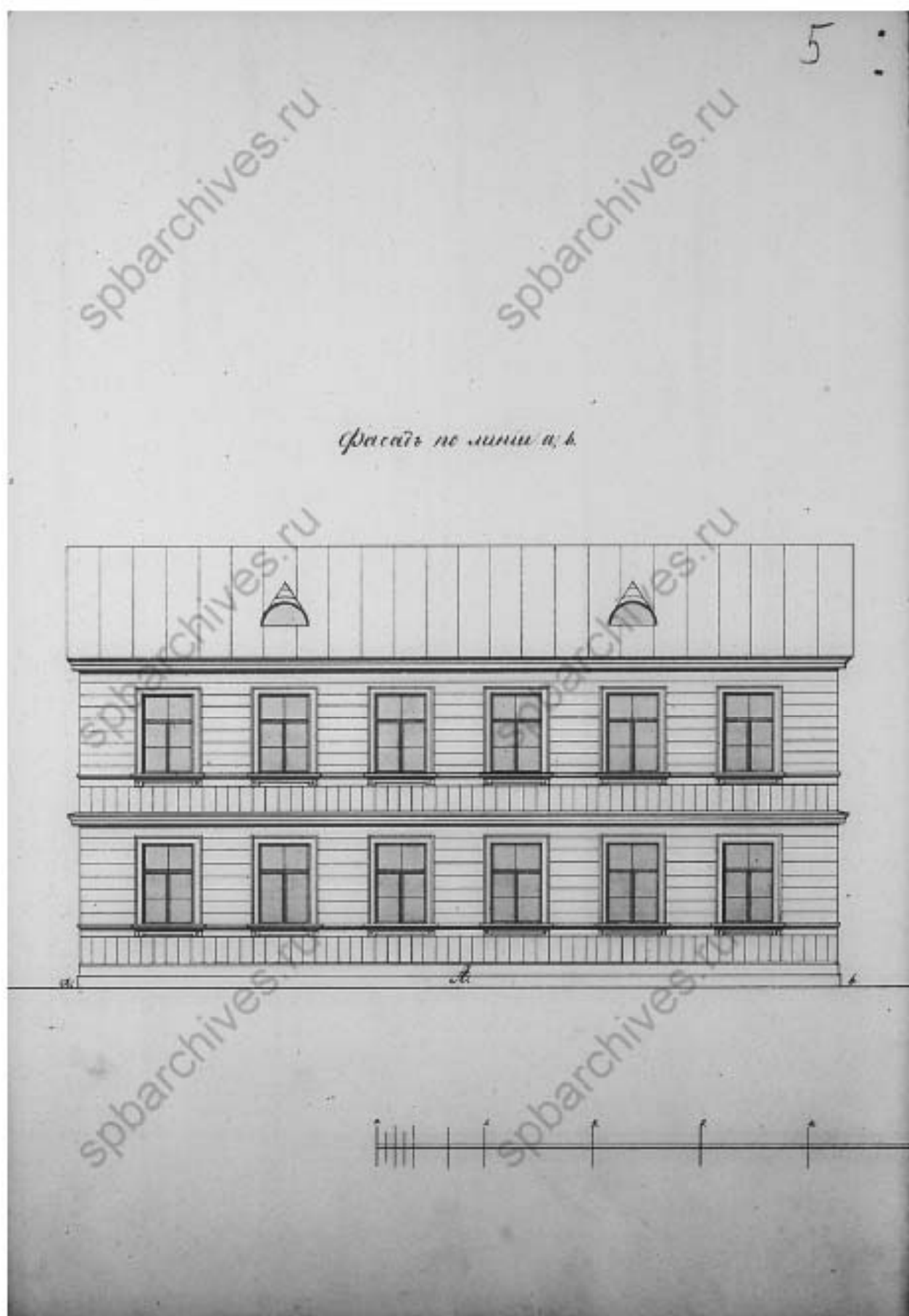
5. Фасад по линии аб. 1871 г. // Источник: ЦГИА СПб Ф.513 Оп.102 Д.9372 Л.5.
