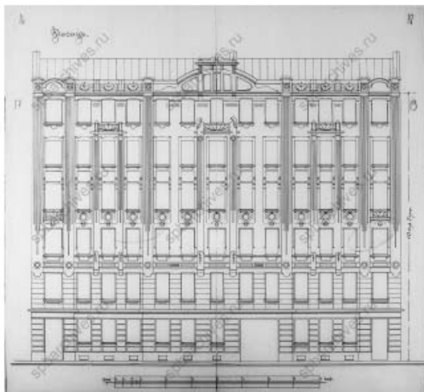
11. Фасад, 1906 г. // Источник: ЦГИА СПб ф.513 Оп.102 Д.9372 Л.16-19.
