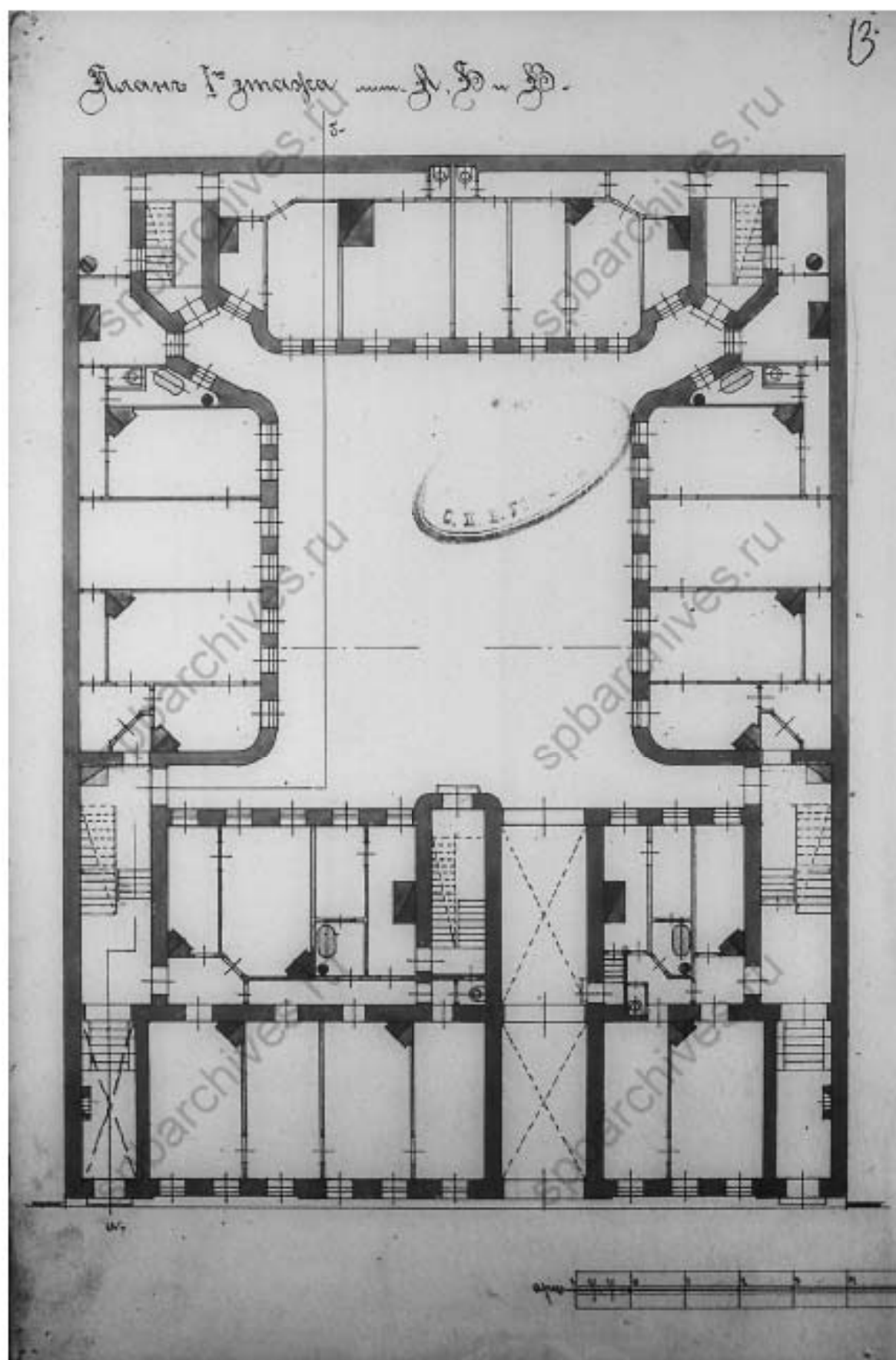
8. План 1-го этажа лит. А, Б и В. 1906 г. // Источник: ЦГИА СПб Ф.513 Оп.102 Д.9372 Л.13.
