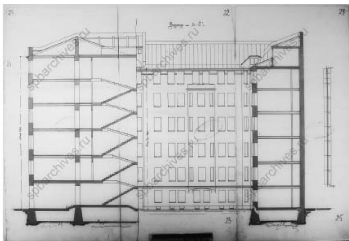
12. Разрез по аб. 1906 г. // Источник: ЦГИА СПб Ф.513 Оп.102 Д.9372 Лл.20-24.
