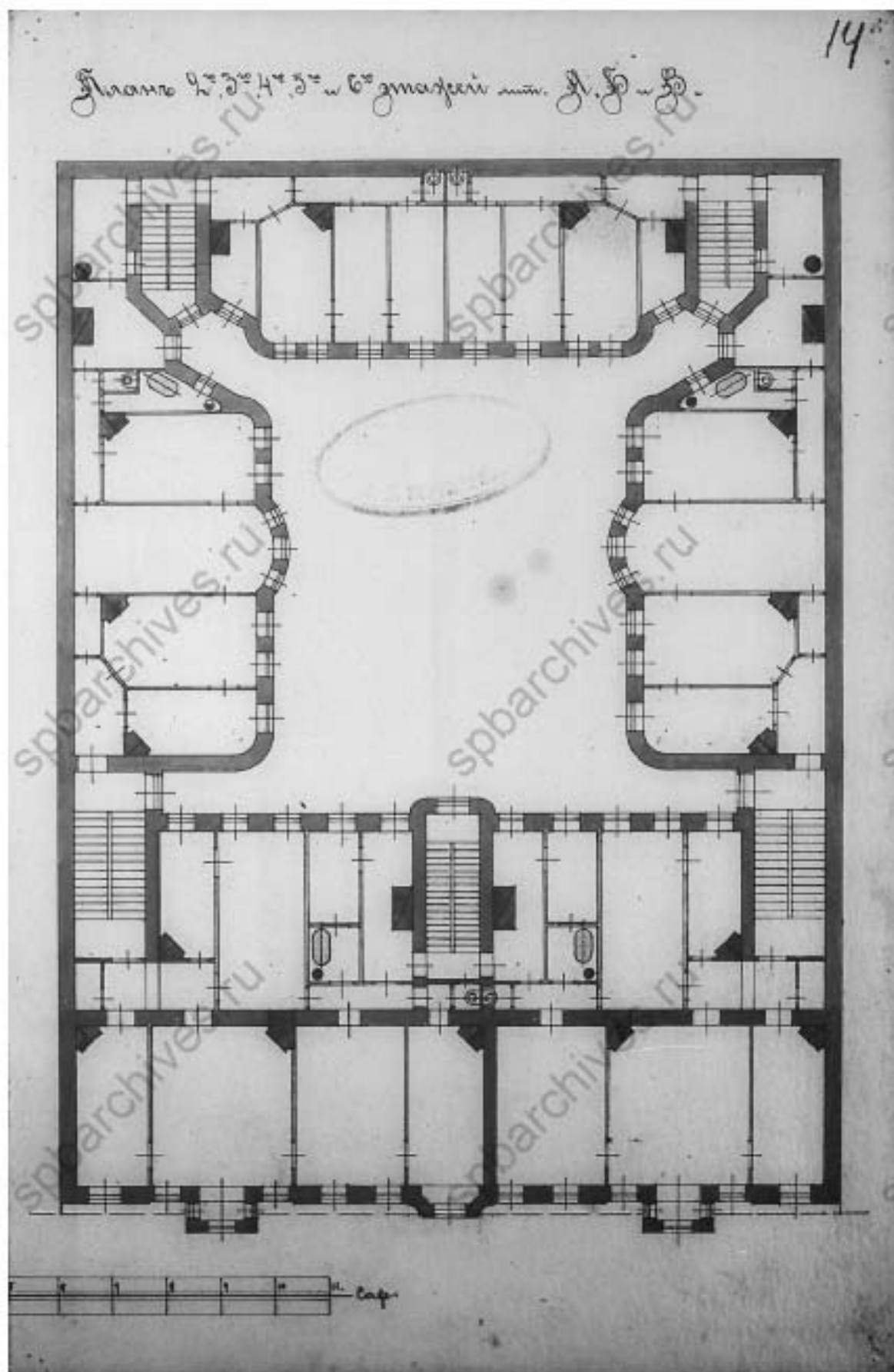
9. План 2-го, 3-го, 4-го, 5-го и 6-го этажей лит. А, Б и В. 1906 г. //
