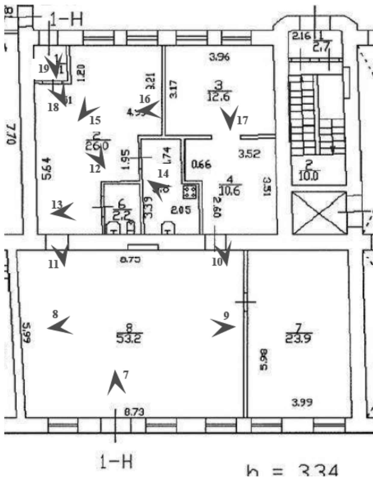
Фрагмент плана 1 этажа Помещение 1-Н
