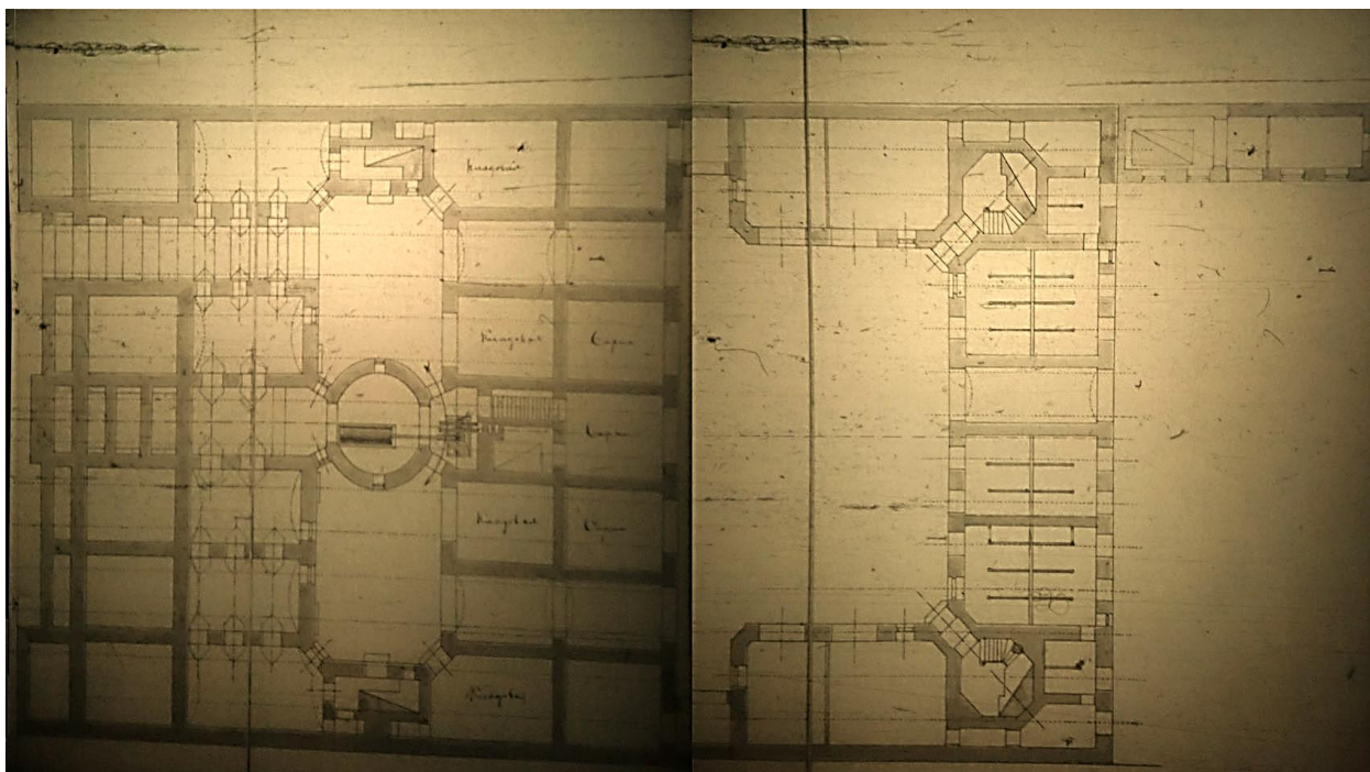
8. План подвала дома потомственного почетного гражданина Григория Елисеева Московской части 2-го уч. по Чернышеву пер. № 14. 1891 г. /ЦГИА СПб. Ф. 513. Оп. 102. Д. 5358. Л. 6-7/
