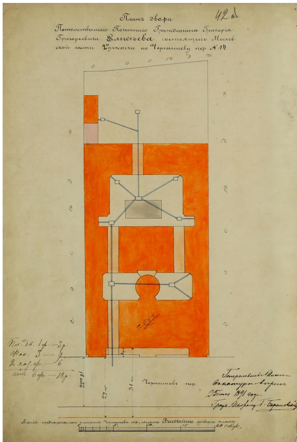
7. План двора потомственного почетного гражданина Григория Елисеева Московской части 2-го уч. по Чернышеву пер. № 14. 1891 г. ЛЦГА СПб. Ф. 513. Оп. 102. Д. 5358. Л. 42 об./
