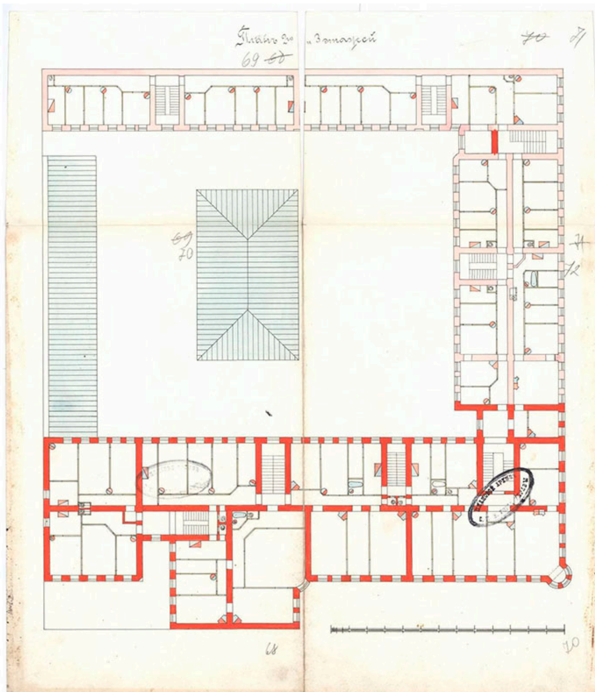
Илл. 22. Проект дома Ф.И. Кривдина. План 2-го и 3-го этажей.
