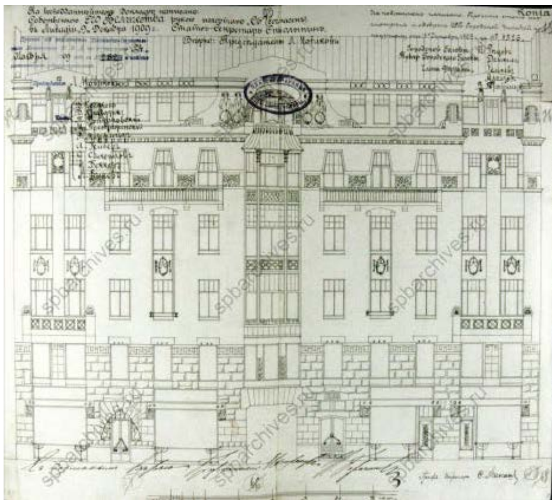
9. Фасад здания по Невскому проспекту. 1909 г. // ЦГИА СПб. Ф. 513. Оп. 102. Д. 4318. Л. 73-76.
