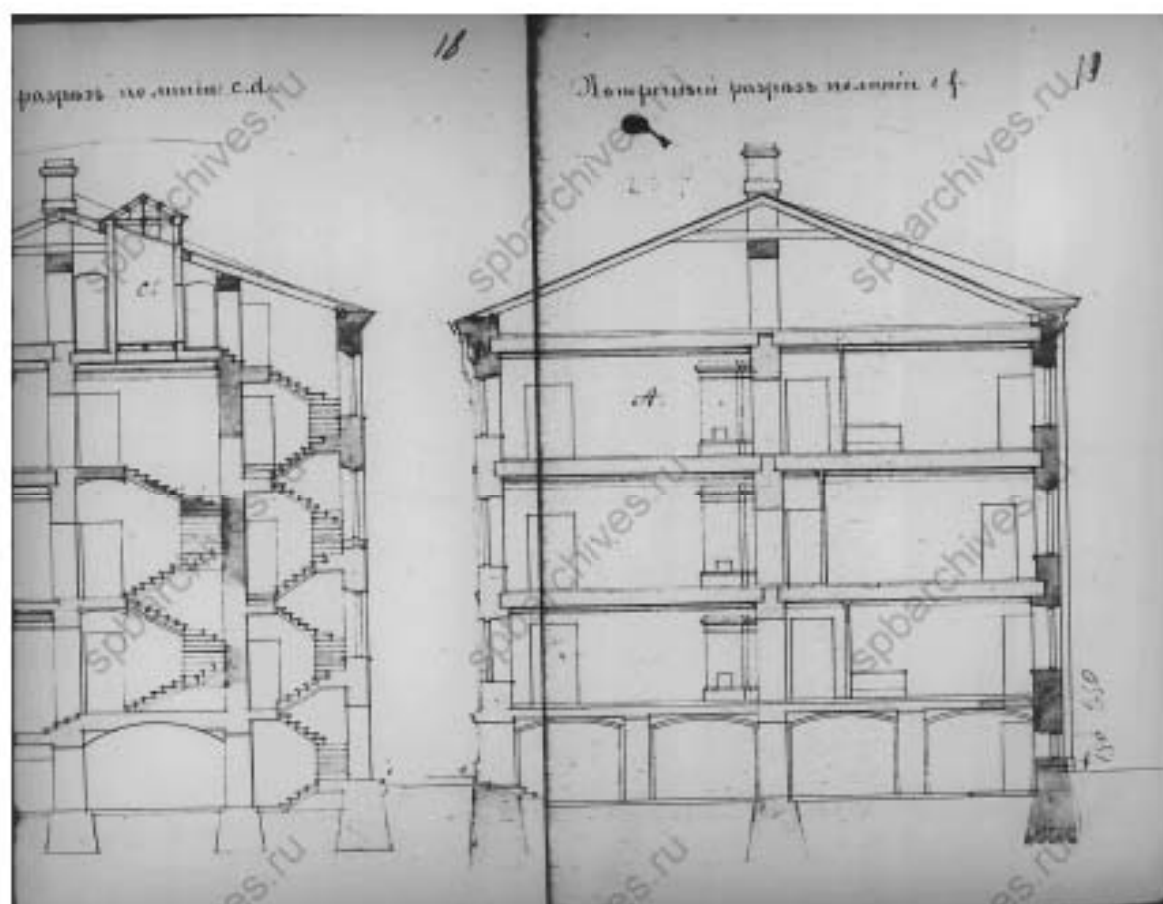
29. Поперечный разрез по линии е.ф. Б.д. // Источник: ЦГИА СПб Ф.513 Оп.102 Д. 1867 Л.19.
