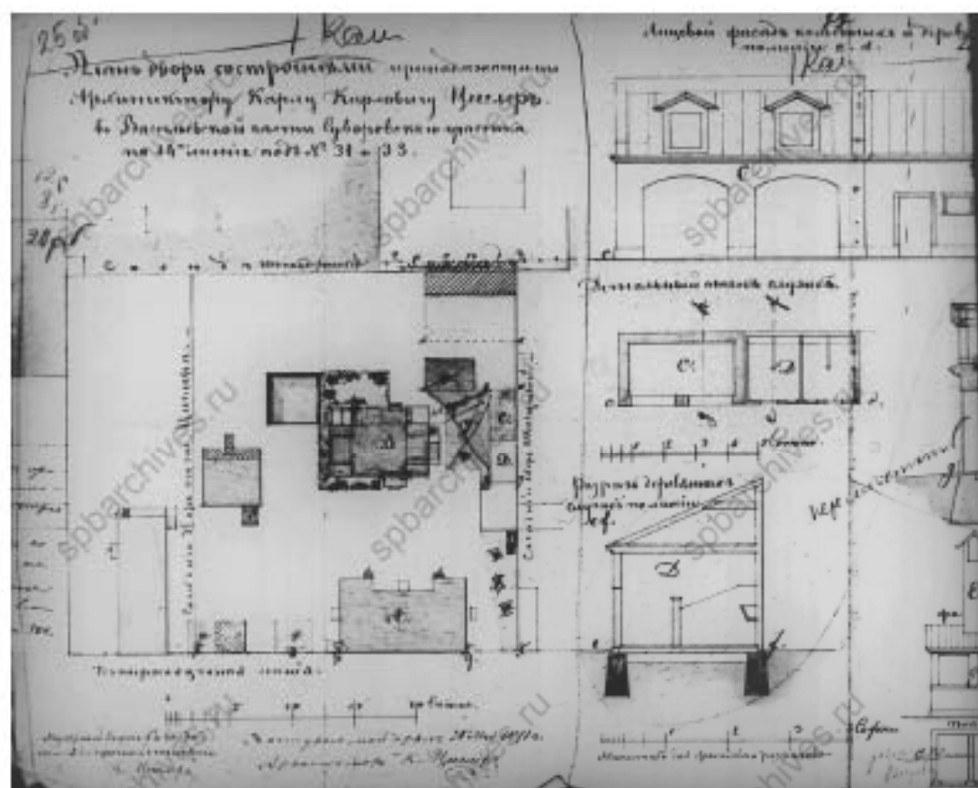
2. План двора со строениями принадлежащими архитектору Карлу Карловичу Циглеру в Васильевской части Суворовского участка по 14-й линии под №31 и 33. 1871 г. Подпись архитектора К.Циглера. // Источник: ЦГИА СПб Ф.513 Оп.102 Д.1866. Л.25об-27.
