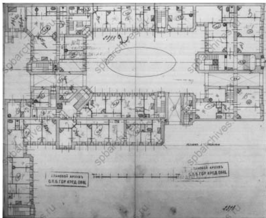
57. План 1-го этажа. Б/д. // Источник: ЦИА СПб Ф.515 Оп.4 Д.2908 Л.2-3.
