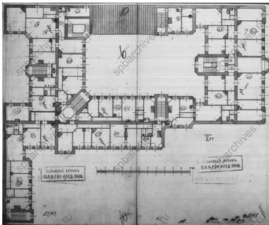
61. План 5-го этажа. Б/д. // Источник: ЦГИА СПб Ф.515 Оп.4 Д.2908 Л.10-11.
