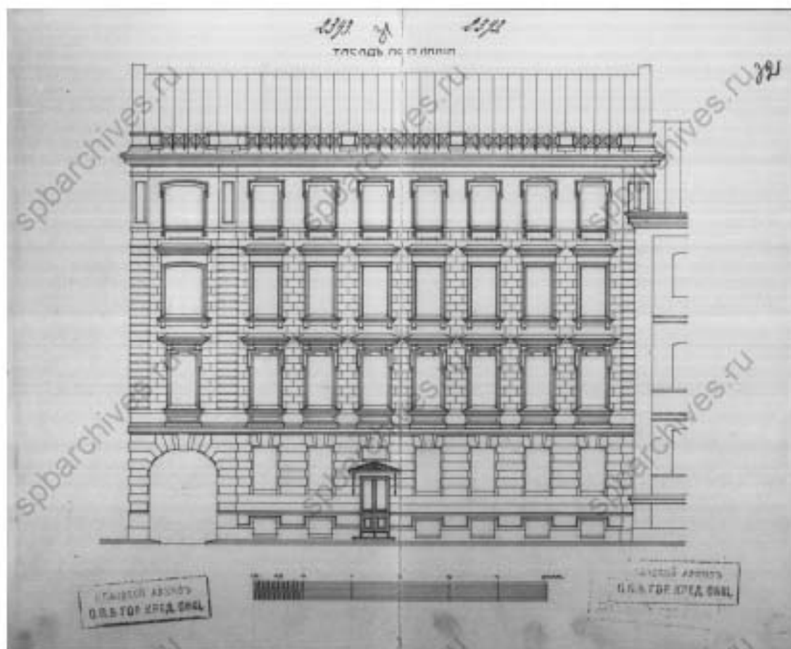
70. Фасад по 14-й линии. Б/д. // Источник6 ЦГИА СПб Ф.515 Оп.4 Д.2908 Л.32.
