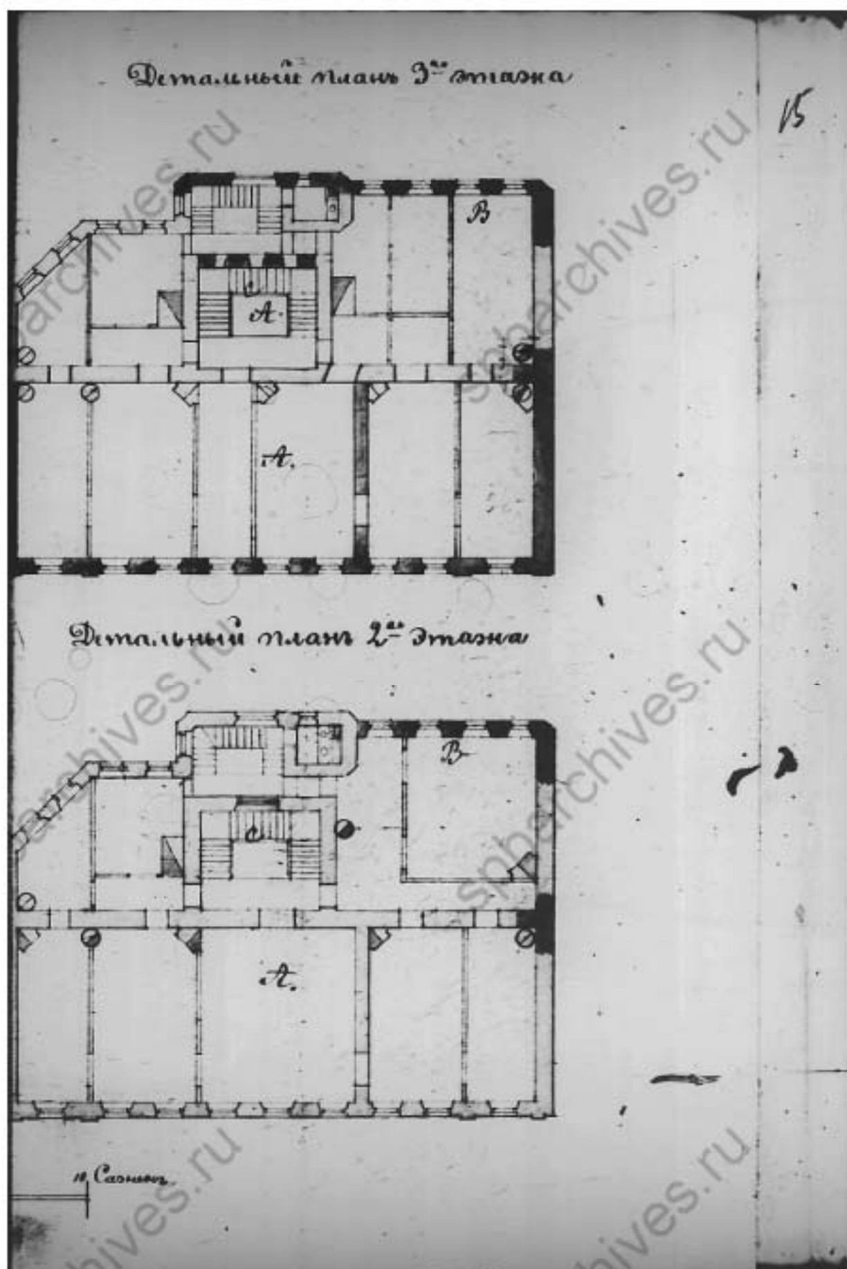
26. Детальный план 3-го этажа. Детальный план 2-го этажа. Б/д. // Источник: ЦГИА СПб Ф.513 Оп.102 Д. 1867 Л.15.
