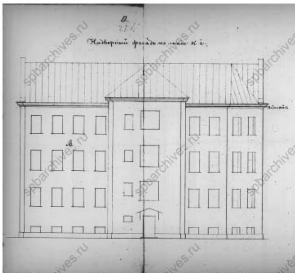
24. Надворный фасад к. Б. д. // Источник: ЦГИА СПб Ф. 513 Оп. 102 Д. 1867 Л. 12.
