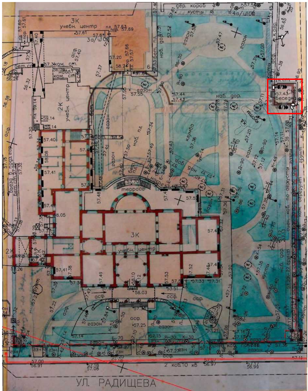
Илл. 19. Совмещённый план топосъёмки 2019 года и проект
