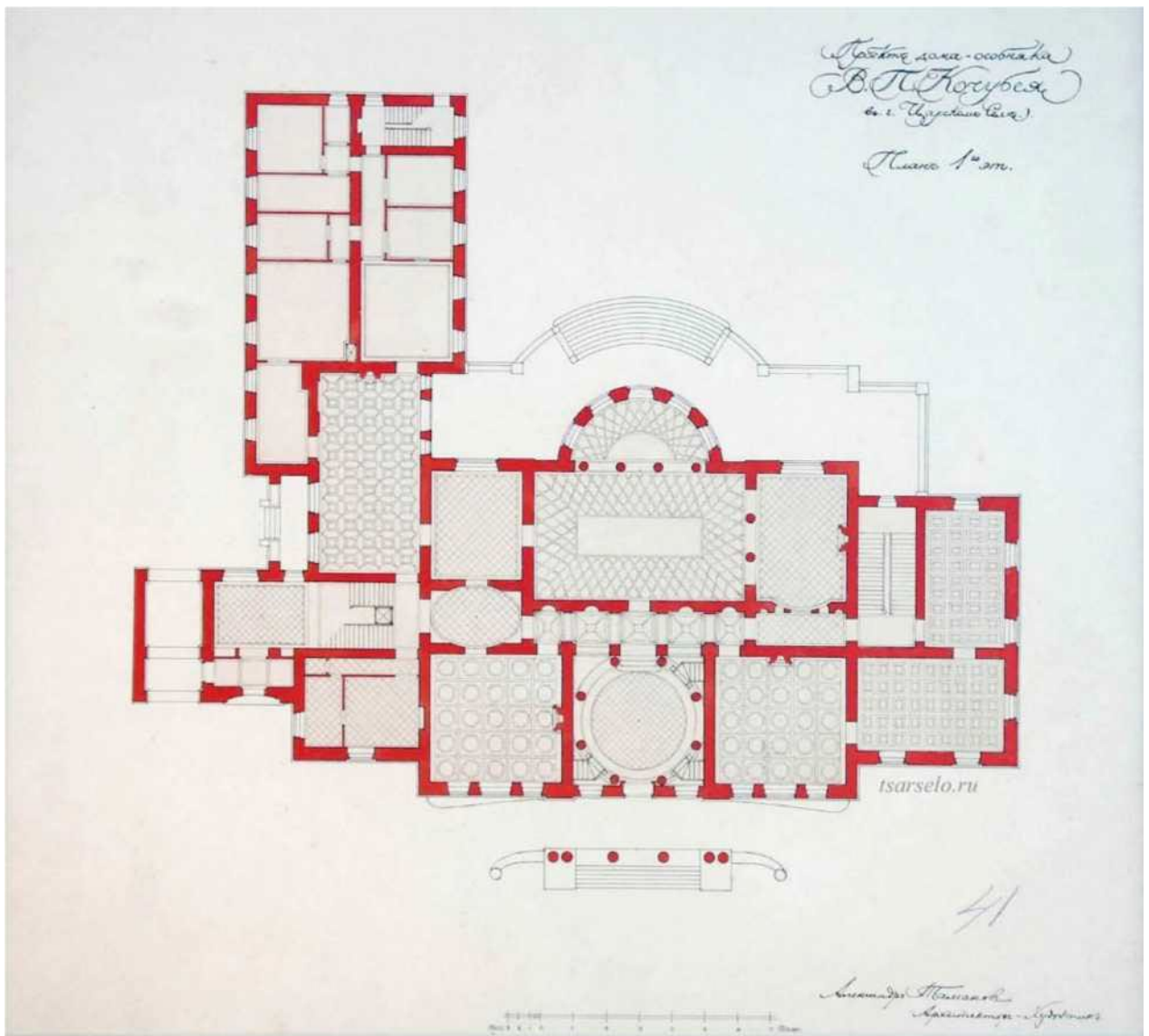
Илл. 7. Таманов Александр. План 1 этажа особняка В.П. Кочубея, 1911 // ГМЗ «Царское Село».
