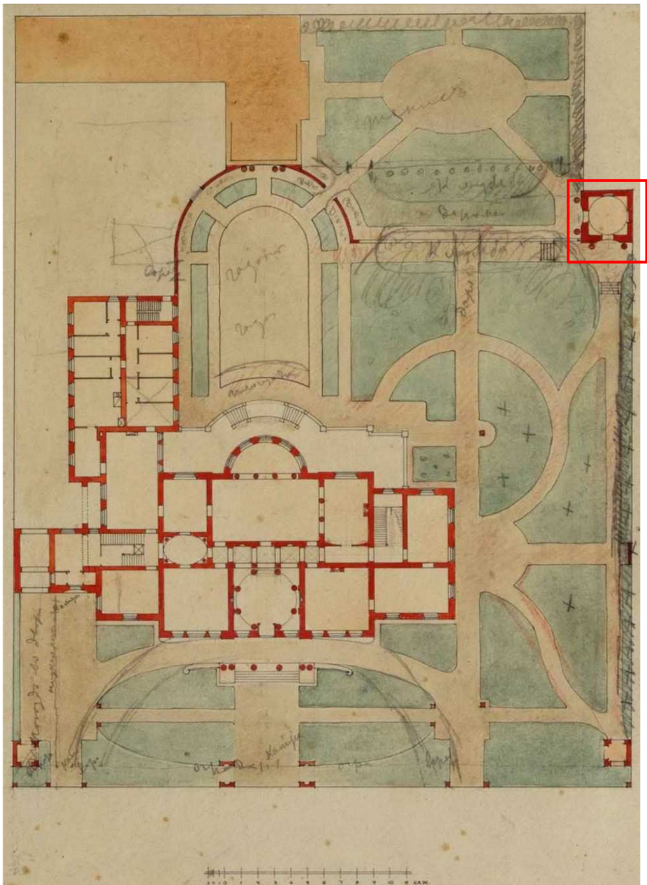
Илл. 9. Проектный план участка. 1911. // ГМЗ «Царское село».
