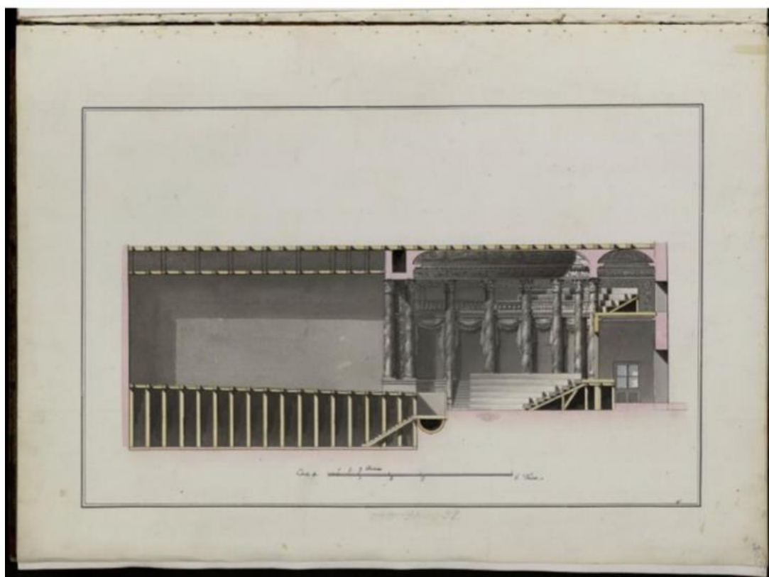
Илл. 27 Руска Л., Тьерри Ж.Э. Проект перестройки театра в Таврическом дворце в Петербурге. 1800-е гг. НИМ РАХ
