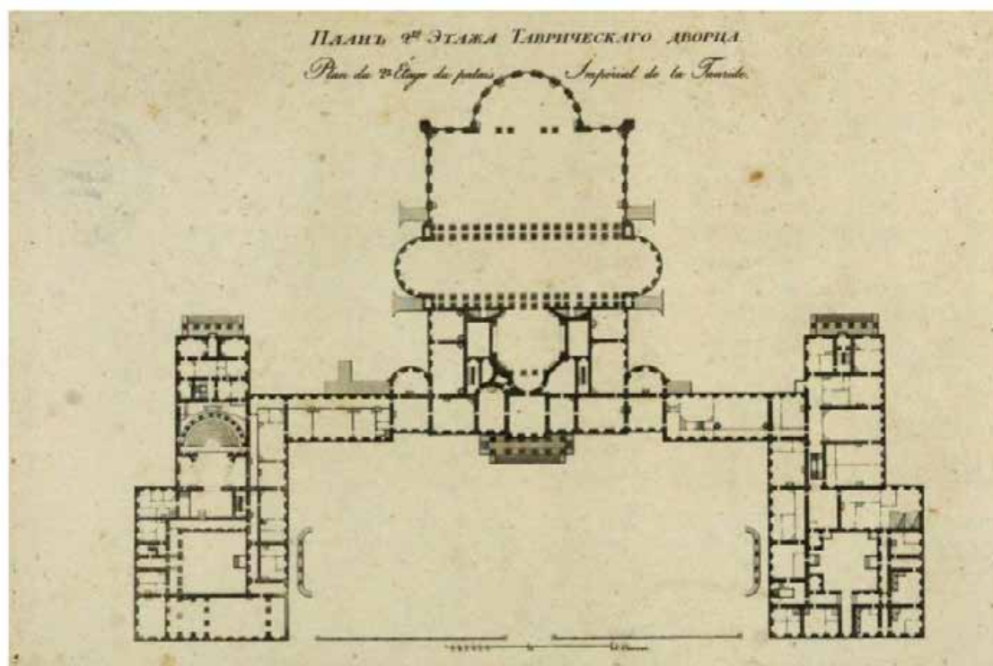
Илл. 45 . Шелковников А.М. План второго этажа Таврического дворца. 1826 г. ГИМ
