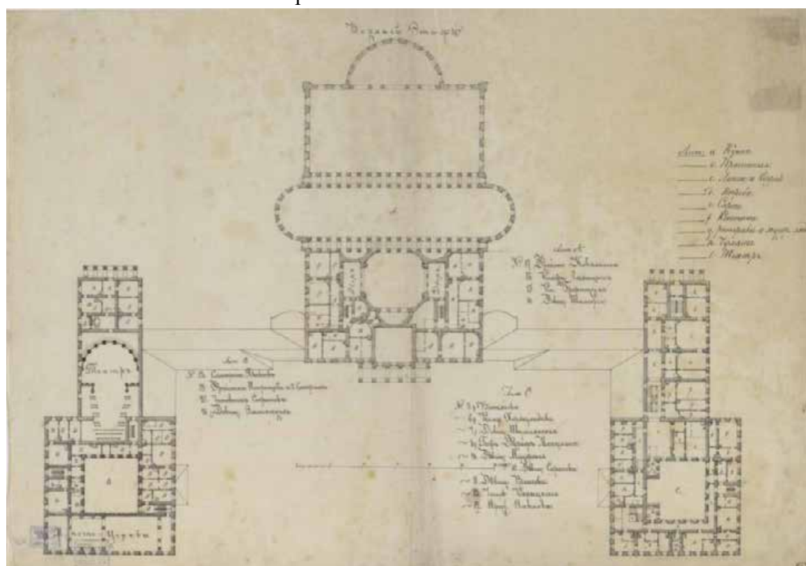
Илл. 32 Неизвестный автор. План Таврического дворца в Петербурге (копия). Второй этаж. XIX в. НИМ РАХ
