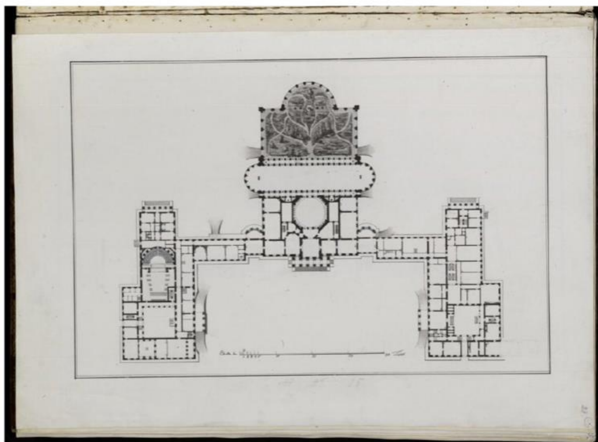
Илл. 24 . Руска Л., Тьерри Ж.Э. Проект перестроек в Таврическом дворце в Петербурге. 1800-е гг. НИМ РАХ
