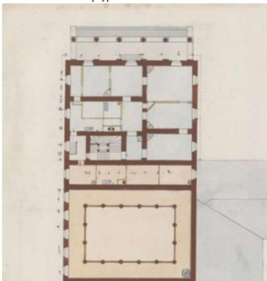
Илл. 57 Неизвестный автор. План второго этажа. Обмер Таврического дворца в Петербурге. 1911 г. НИМ РАХ. Фрагмент
