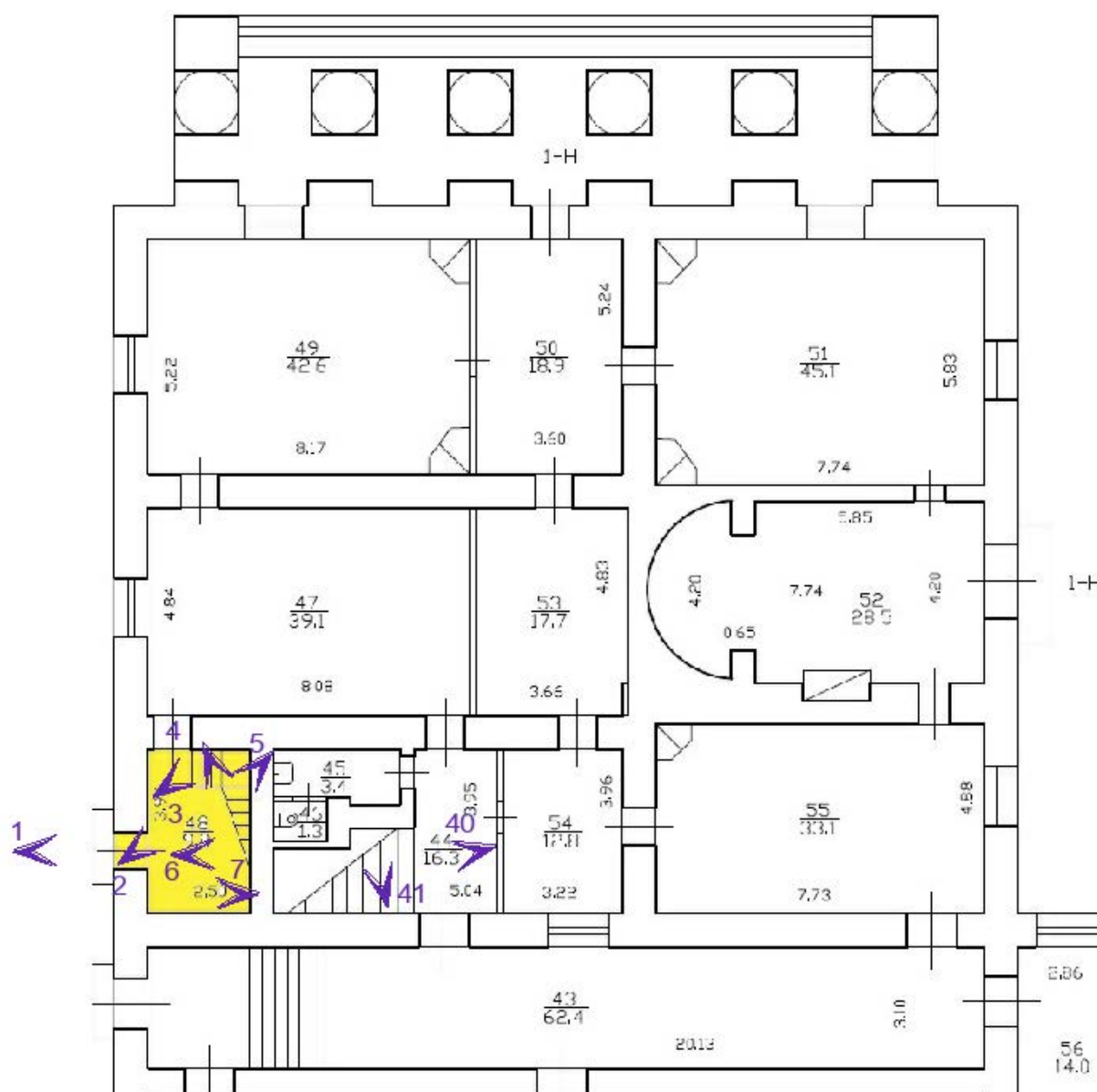
Рисунок 1. Схема фотофиксации 1 этажа.
