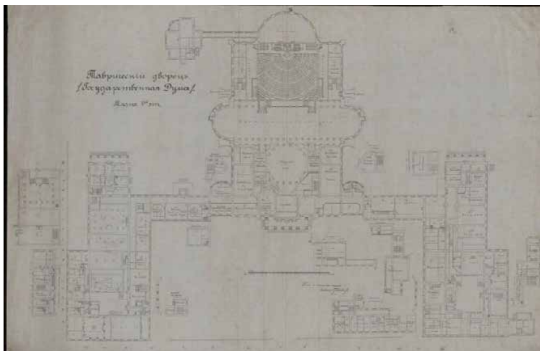
Илл. 58 Неизвестный автор. Обмер Таврического дворца в Петербурге. План первого этажа. 1911 г. НИМ РАХ
