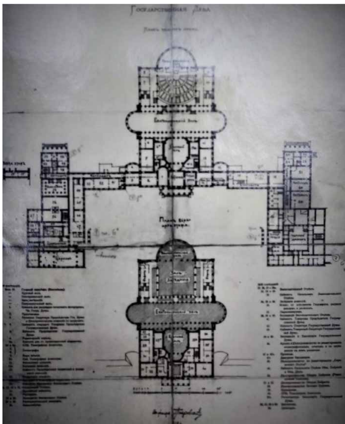
Илл. 62 . Инженер Пиотровский План Государственной думы. 1912 г.
