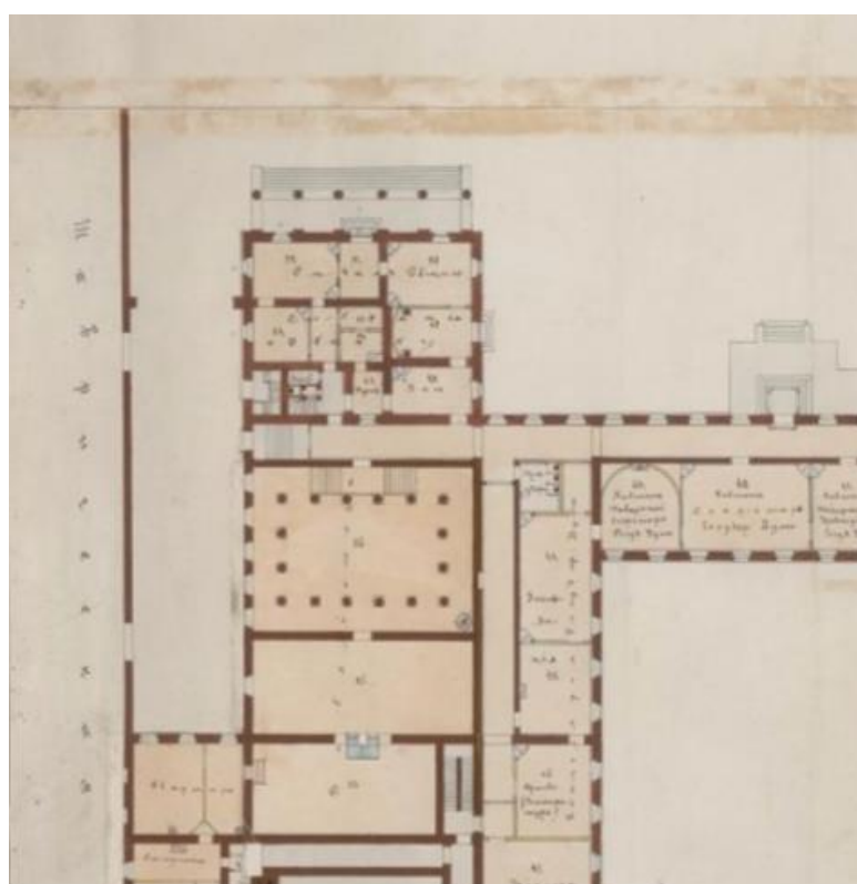
Илл. 55 Неизвестный автор. План первого этажа. Обмер Таврического дворца в Петербурге. 1911 г. НИМ РАХ. Фрагмент.
