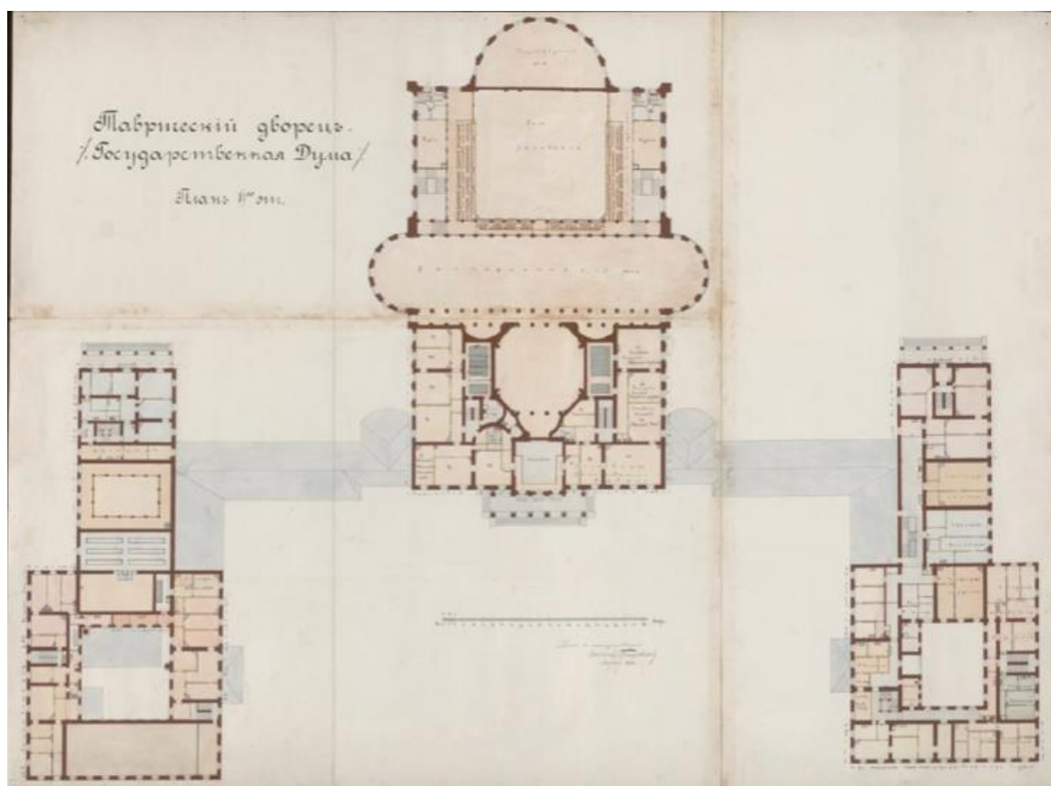
Илл. 56 Неизвестный автор. План второго этажа. Обмер Таврического дворца в Петербурге. 1911 г. НИМ РАХ
