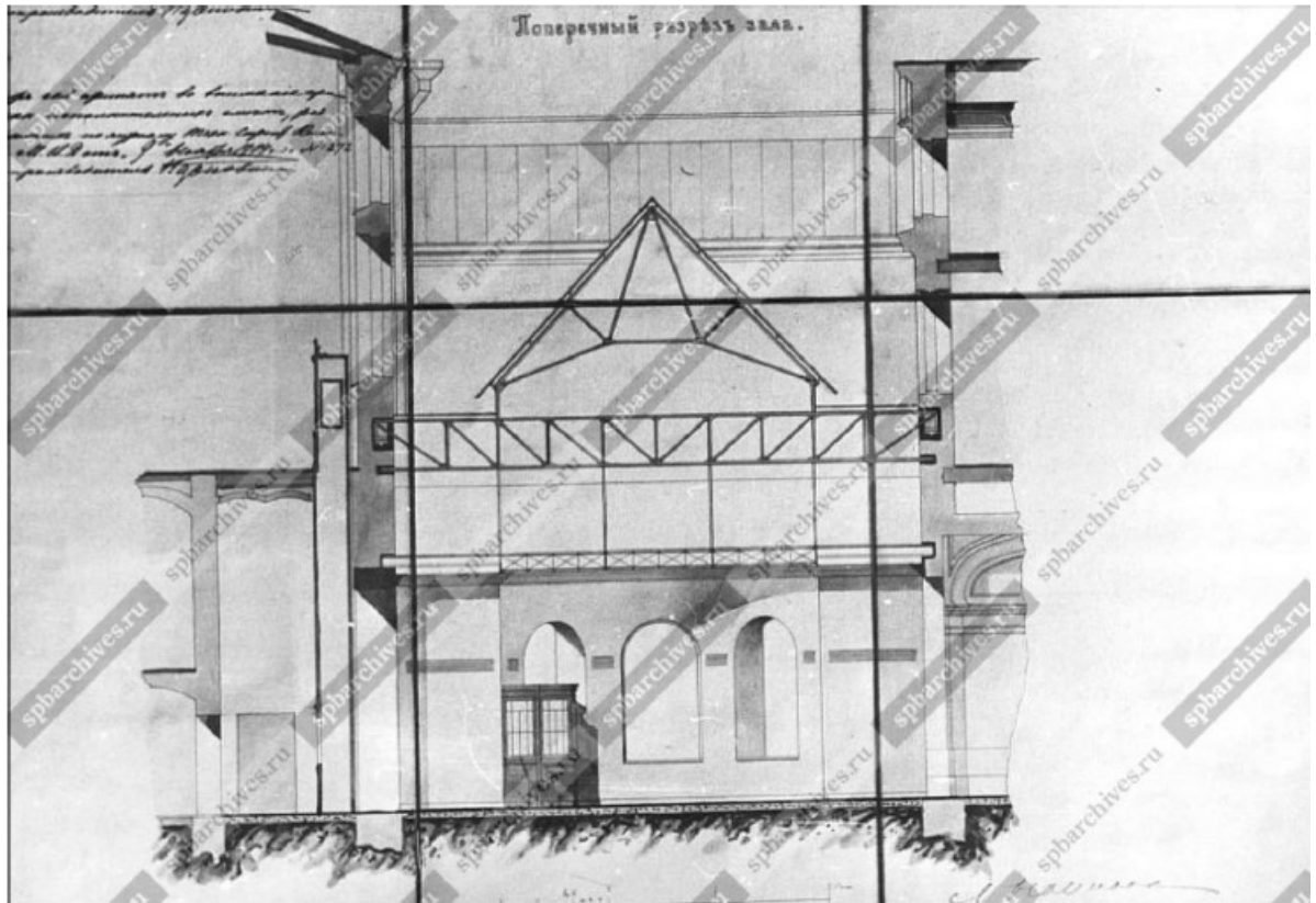
Илл. 20. Чертеж поперечного разреза зала. 1903 г. ЦГАКФФД СПб. Фотодокумент А 5628.
