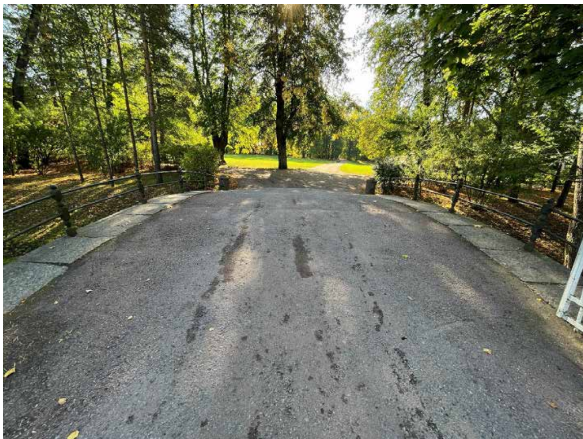
Фото 2. Однопролётный каменный мост с каменными устоями и цилиндрическим сводом. Общий вид с северной стороны. Дата фотофиксации: 29.08.24
