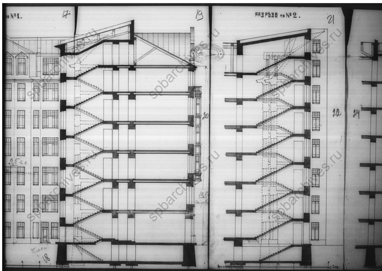
15. Разрез по № 2. Чертежи дома на участке, принадлежавшем Г.Г.Подгорному, М.И.Грибкову по Зверинской ул., 31. ЦГИА СПб. Фонд 513. Опись 102. Дело 7681. 1873–1913 гг.
