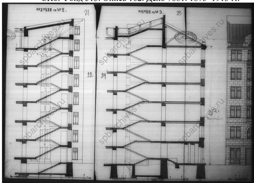
16. Разрез по № 3. Чертежи дома на участке, принадлежавшем Г.Г.Подгорному, М.И.Грибкову по Зверинской ул., 31. ЦГИА СПб. Фонд 513. Опись 102. Дело 7681. 1873–1913 гг.
