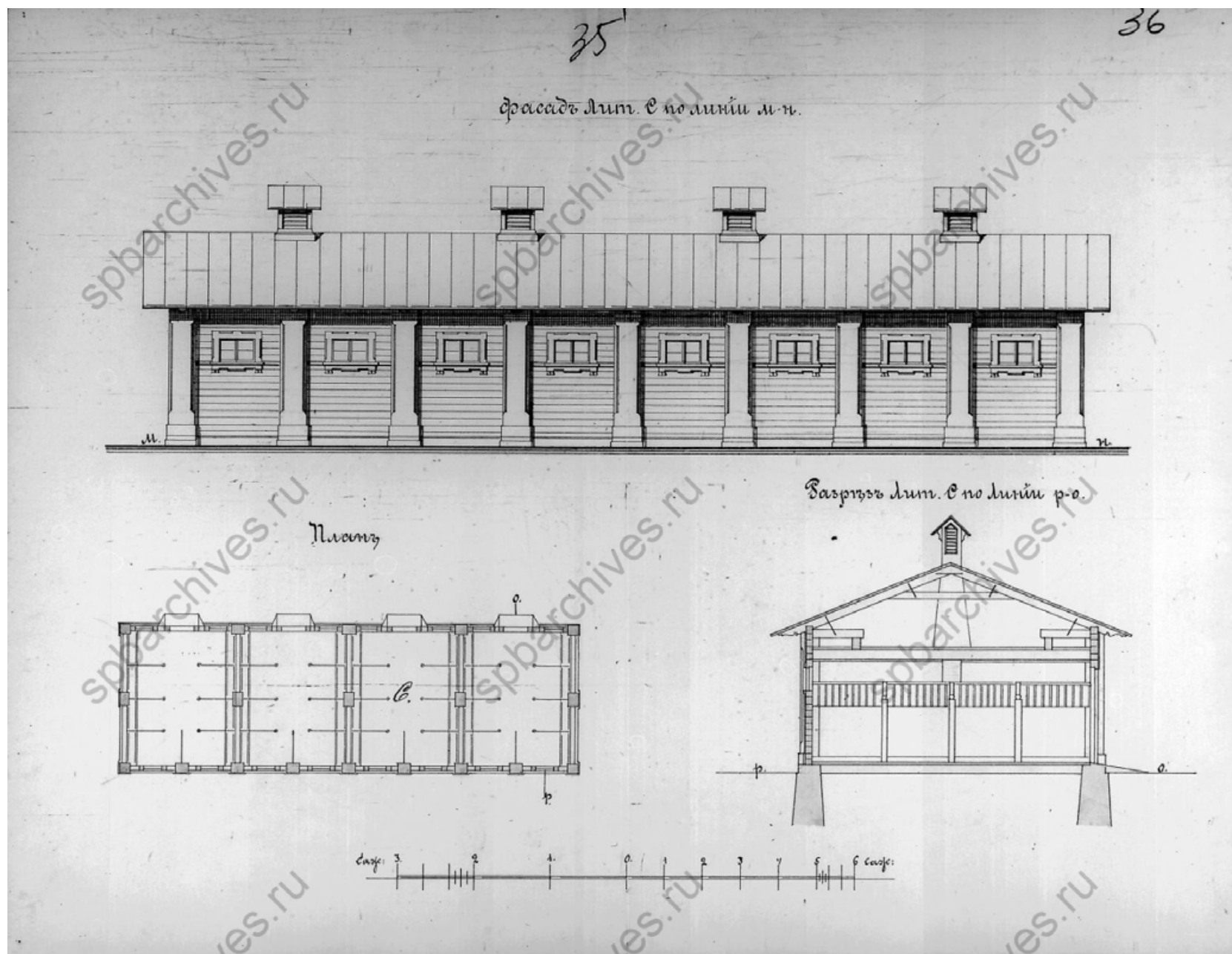
27. Фасад лит. С по линии mn. Б/д. // Источник: ЦГИА СПб. Ф. 513. Оп. 102. Д. 564. Л.35-36.
