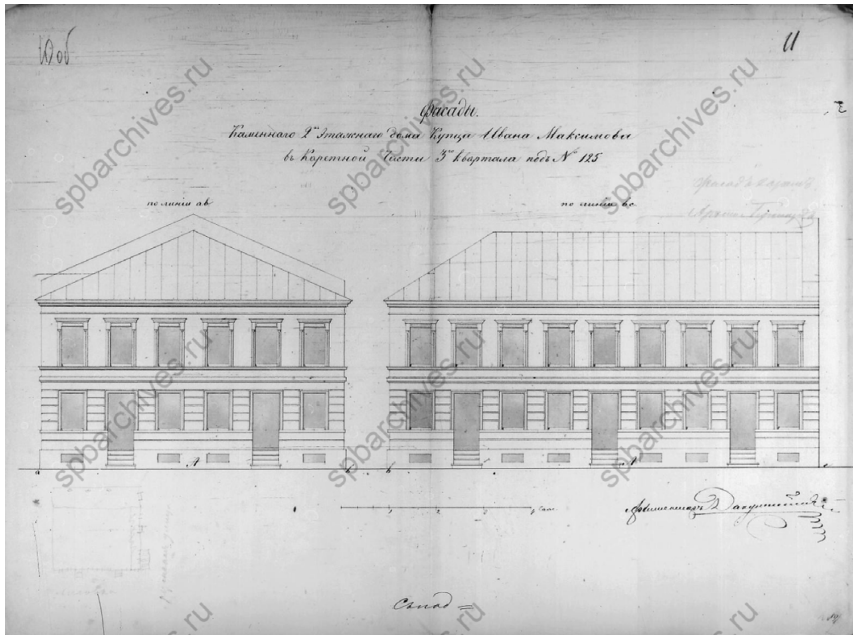
9. Фасады каменного 2-этажного дома купца Ивана Максимова в Каретной части 3-го квартала под №125. Б/д. // Источник: ЦГИА СПб. Ф. 513. Оп. 102. Д. 564. Л. 10об-11.
