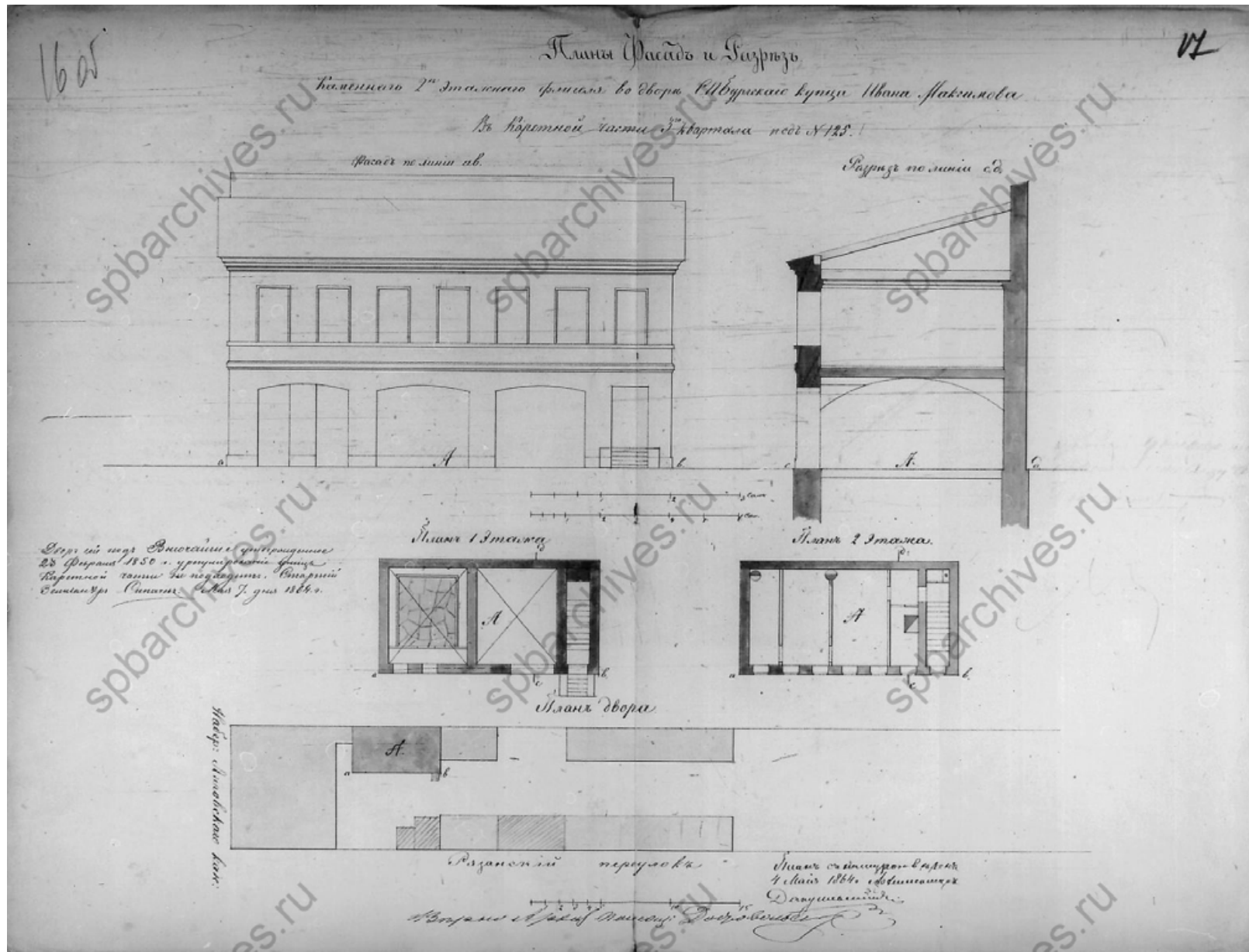
12. Планы, фасад и разрез каменного 2-хэтажного флигеля во дворе СПбургского купца Ивана Максимова в Каретной части 3-го квартала под №125. 1864 г. // Источник: ЦГИА СПб. Ф. 513. Оп. 102. Д. 564. Л. 16об-17.
