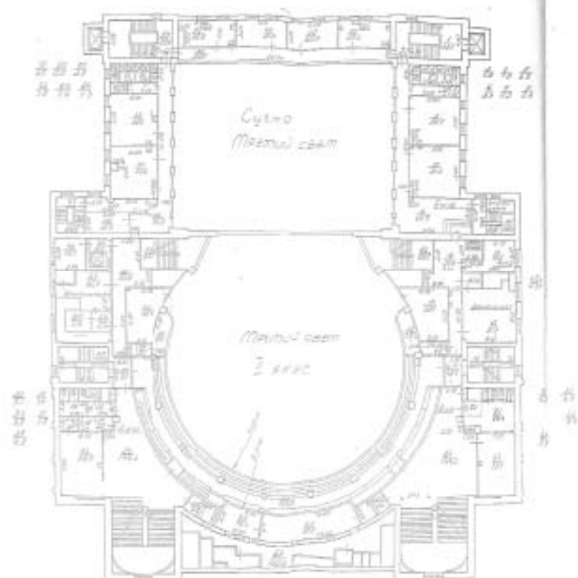
План 4-этажа
