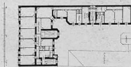
Домъ И. И. Боргмана, Съезженская, 4, С.-Петербургъ. Г. Д. ГРИММЪ, академ. архит. С. П. Бургъ.
