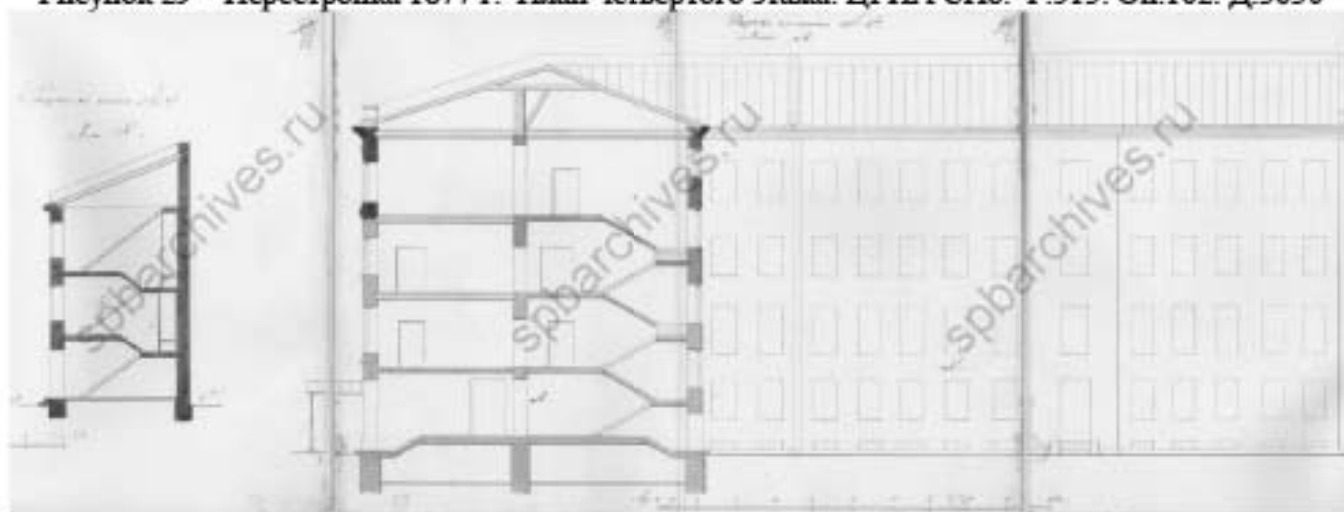
Рисунок 30 – Перестройка 1877 г. Разрезы. ЦГИА СПб. Ф.513. Оп.102. Д.3630
