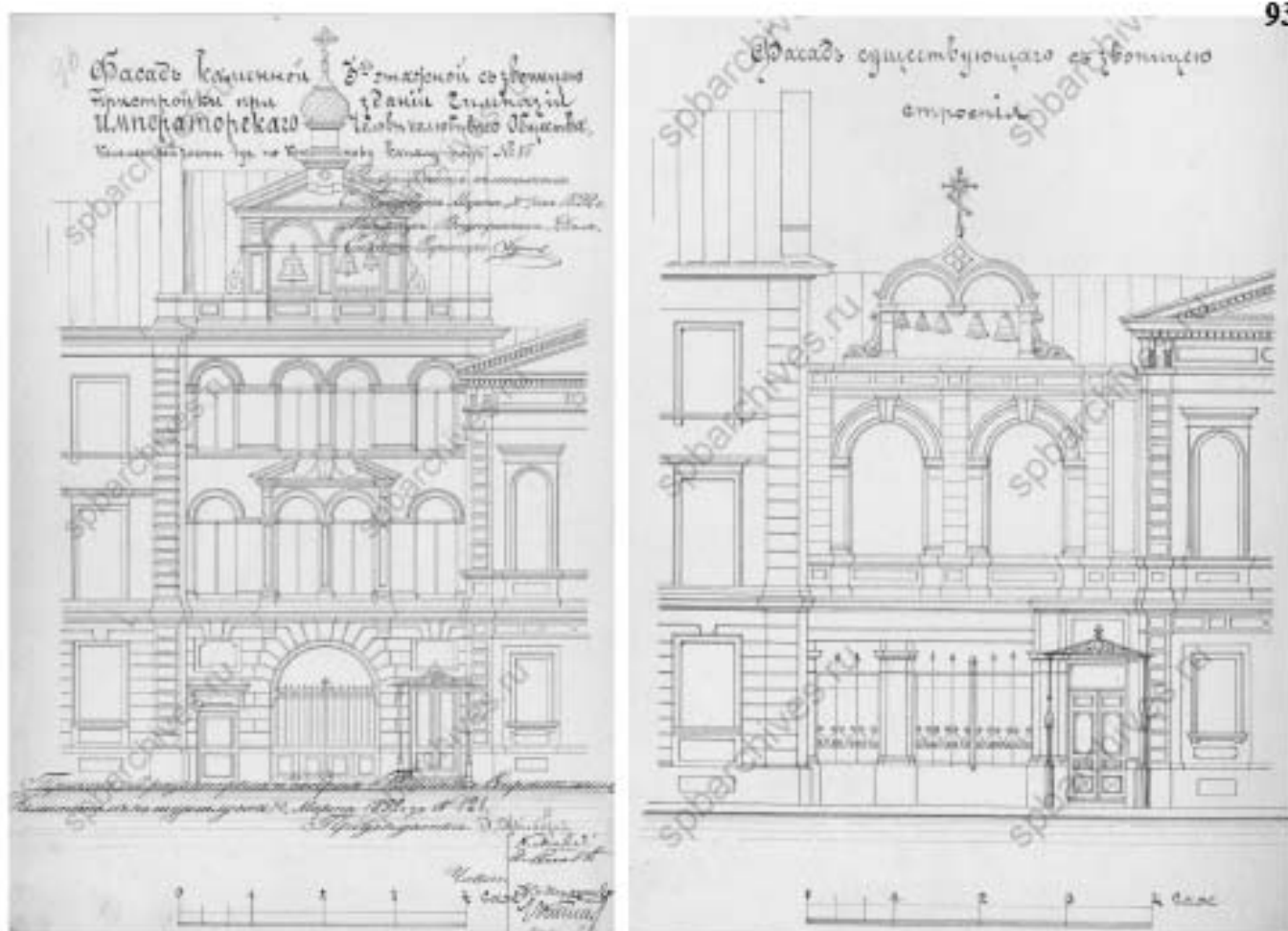
Рисунок 49 – Фасады каменной звонницы, 1892 г. ЦГИА СПб. Ф.513. Оп.102. Д.3630
