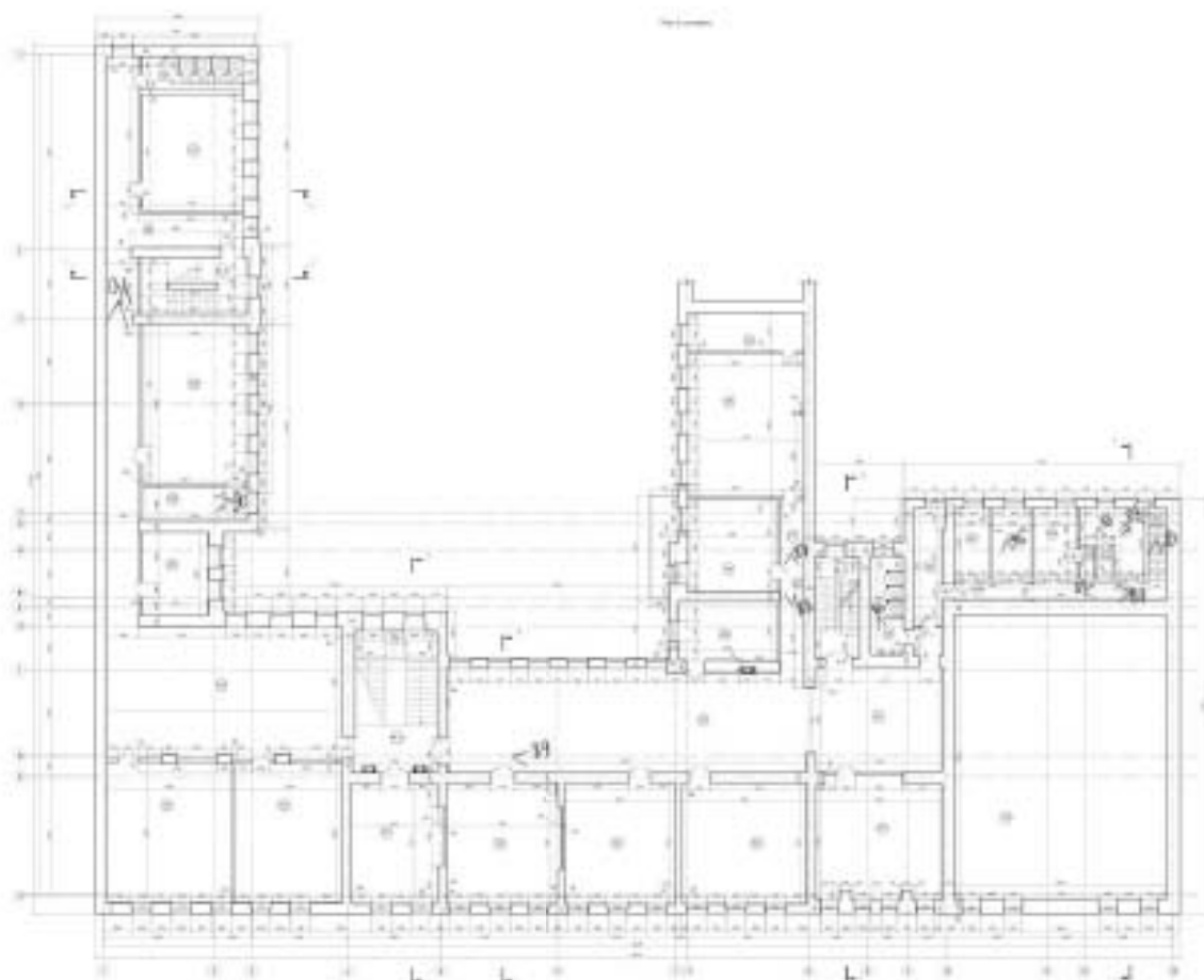
Рис. 2. Схема фотофиксации в уровне 1 этажа.
