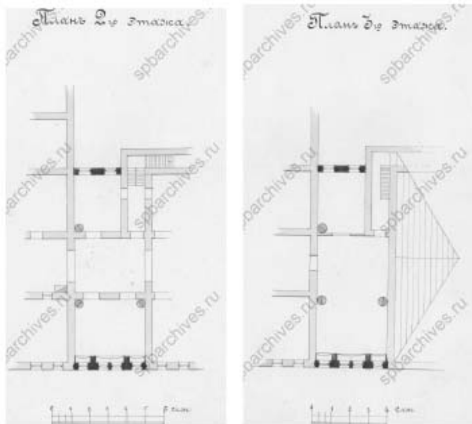
Рисунок 47 – Планы 2,3 этажей, 1892 г. ЦГИА СПб. Ф.513. Оп.102. Д.3630
