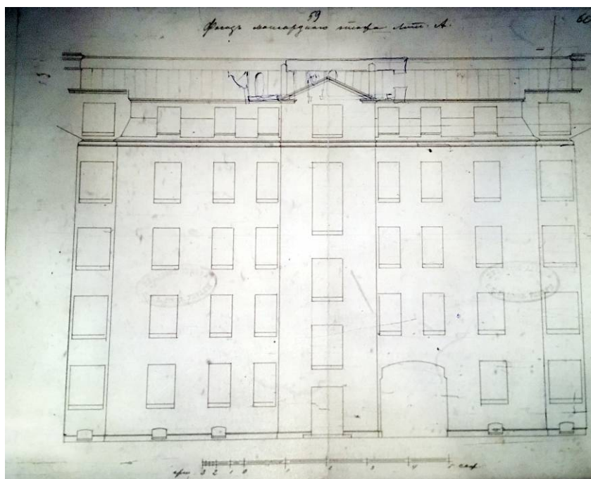
19. План надстройки мансарды. Фасад литера А. 1902. ЦГИА СПб. Ф. 513. Оп. 102. Д. 7602. ЛЛ. 59, 60.
