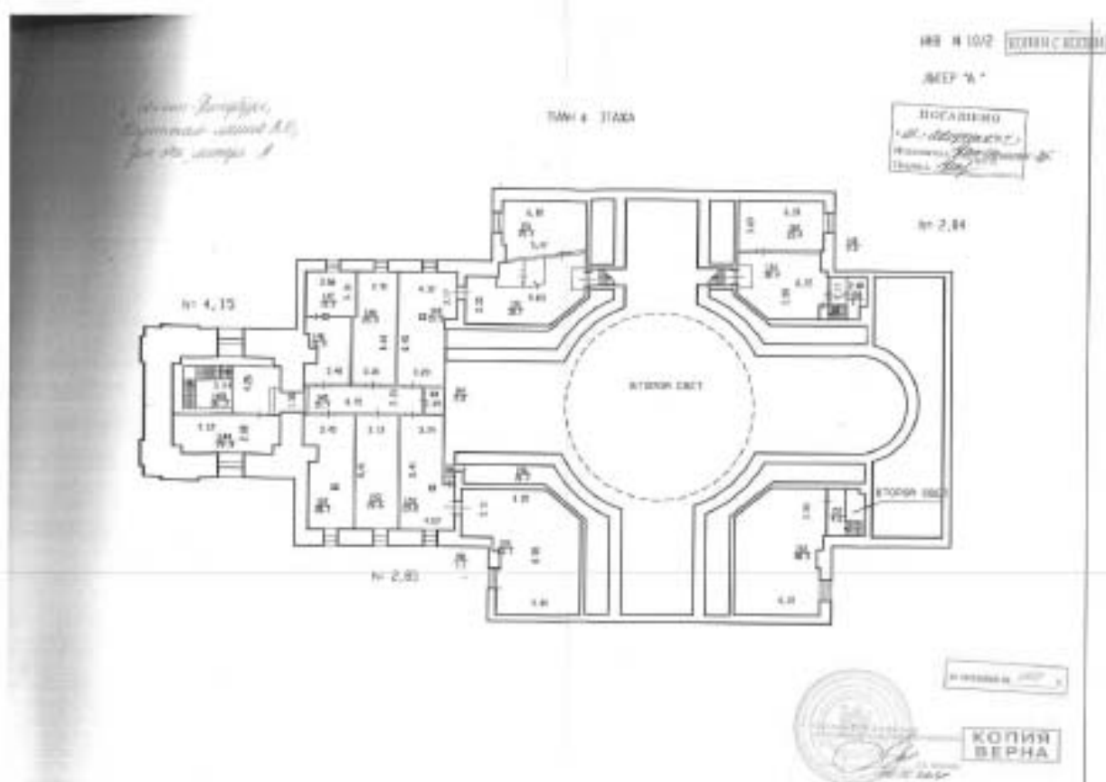
Илл. 18. План 4 этажа по состоянию на 1951 г.
