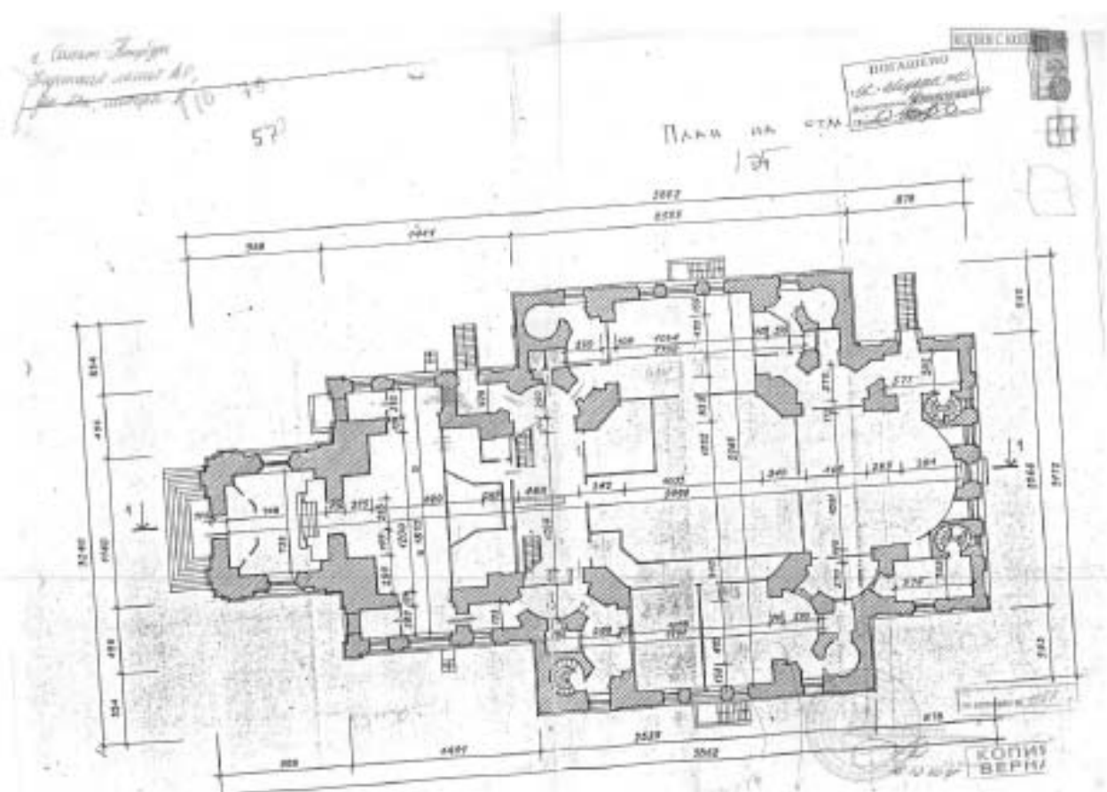
Илл. 15. План 1 этажа по состоянию на 1951 г.
