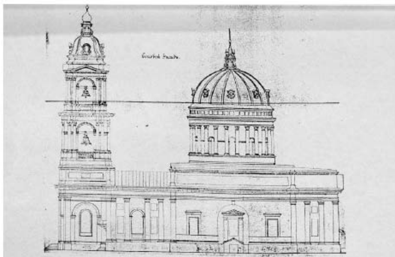
Илл. 5. Проектный чертёж (южный фасад) Церковь Св. Великомученицы Екатерины. Арх. Л.Л. Бонштедт, В.А. Болотов. 1862 г.
