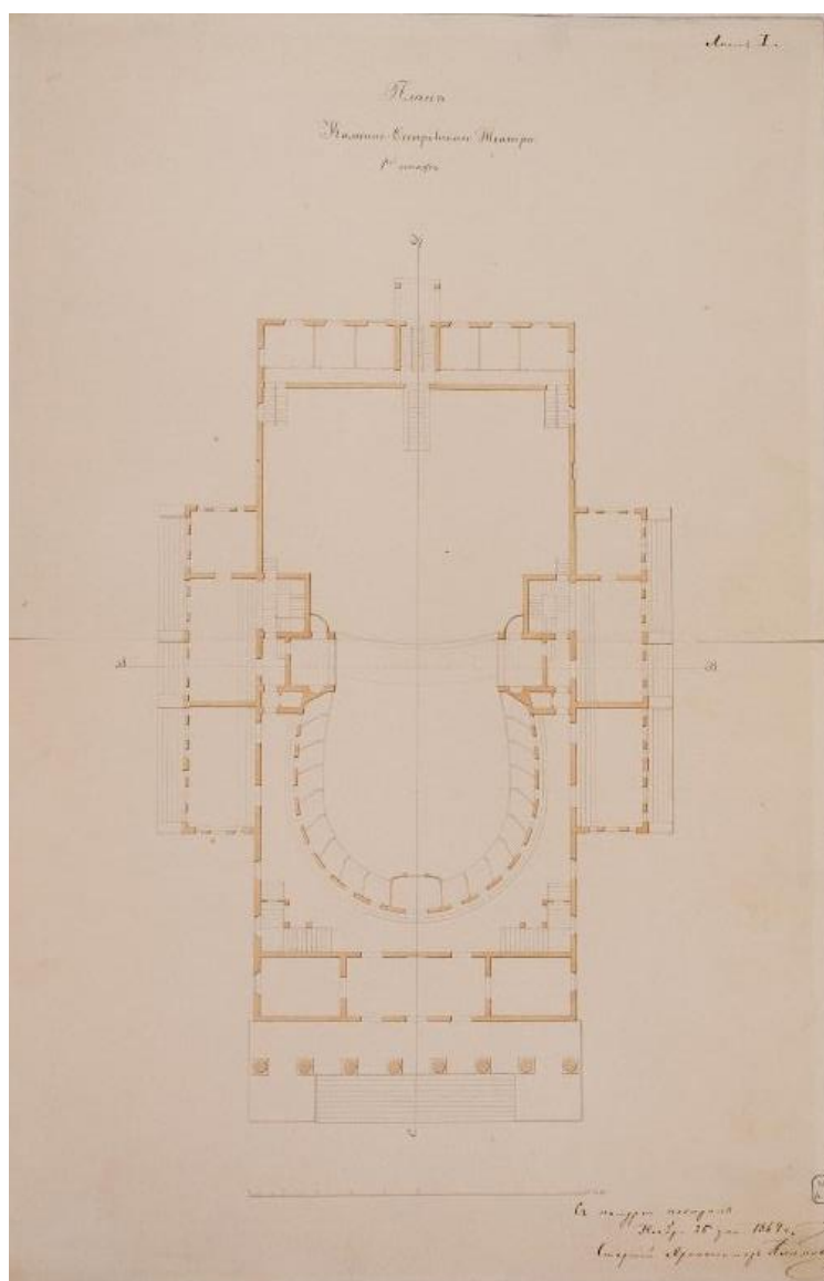
15. Арх. И.И. Климов. Обмер Каменноостровского театра в Санкт-Петербурге (бумага, тушь, заливка акварелью). 1864 г. НИМ РАХ КП-49/21.
