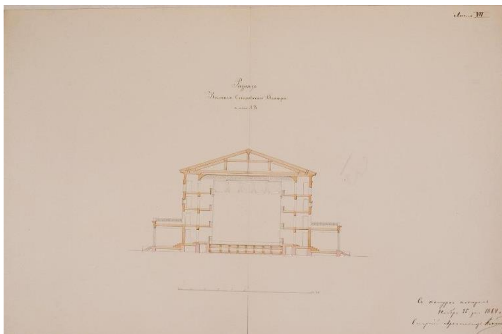
13. Арх. И.И. Климов. Обмер Каменноостровского театра в Санкт-Петербурге (бумага, тушь, заливка акварелью). 1864 г. НИМ РАХ КП-49/27.
