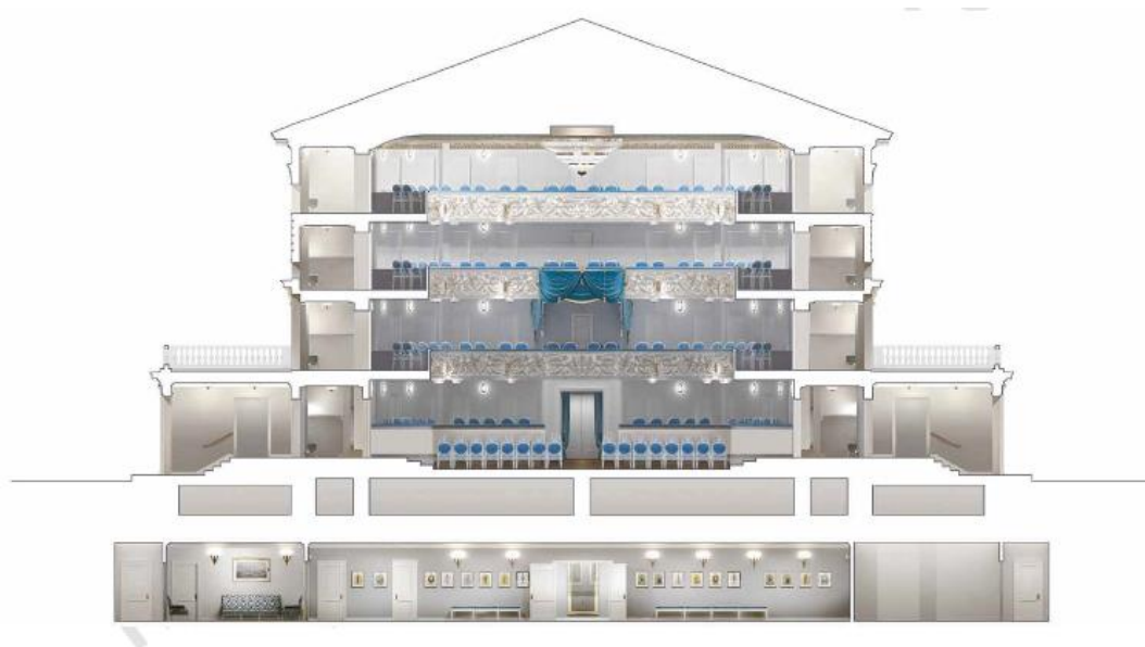
58. Каменноостровский театр. Проект реставрации приспособления для современного использования. 2007-2011 гг. Поперечный разрез по зрительному залу. Опубликовано в: Дементьева В.А., Рахманов В.С., Шашкин А.Г., Бурыгин В.А. Каменноостровский театр. Синтез достижений реставрации и геотехники». (авторы:). СПб., 2014.
