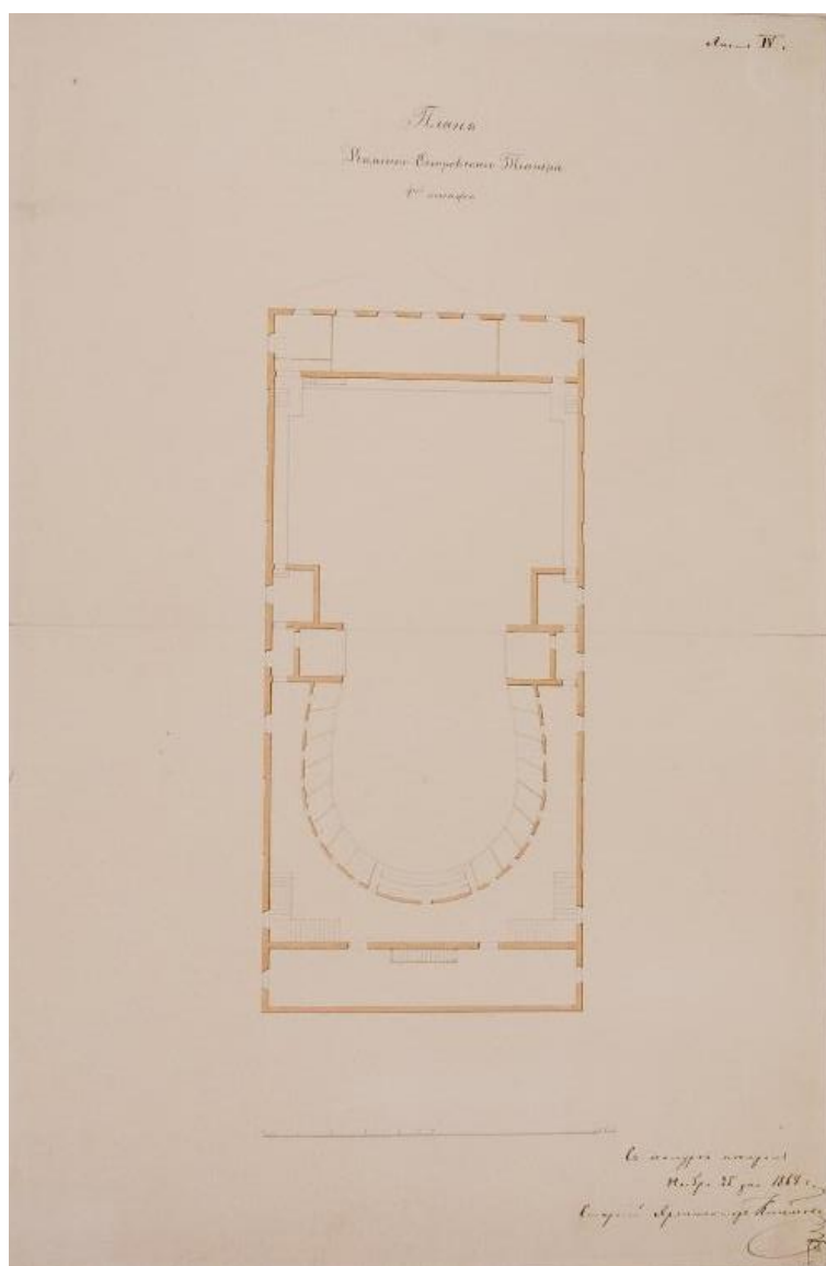
18. Арх. И.И. Климов. Обмер Каменноостровского театра в Санкт-Петербурге (бумага, тушь, заливка акварелью). 1864 г. НИМ РАХ КП-49/24.
