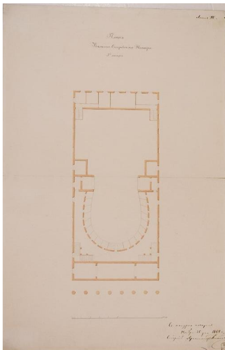
17. Арх. И.И. Климов. Обмер Каменноостровского театра в Санкт-Петербурге (бумага, тушь, заливка акварелью). 1864 г. НИМ РАХ КП-49/23.
