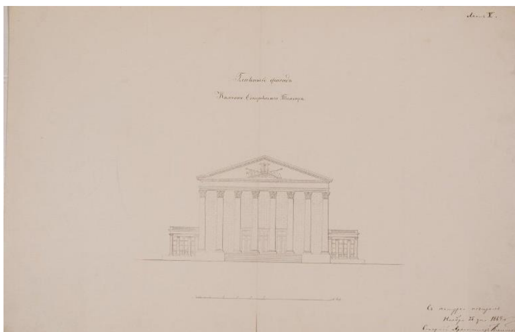
11. Арх. И.И. Климов. Обмер Каменноостровского театра в Санкт-Петербурге (бумага, тушь, заливка акварелью). 1864 г. НИМ РАХ КП-49/25.
