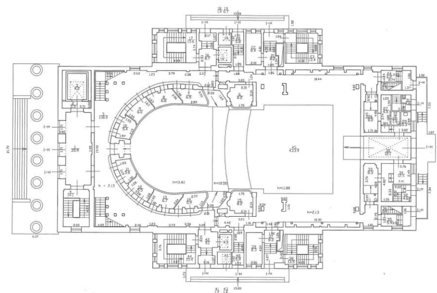
План 1 этажа
