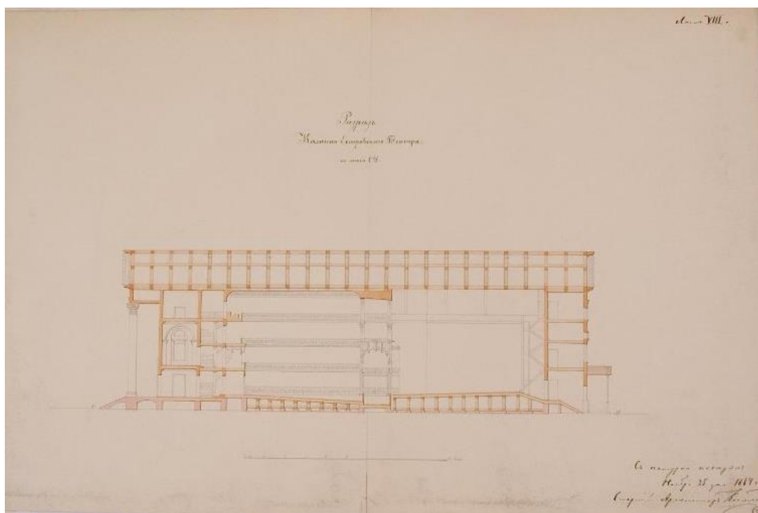
14. Арх. И.И. Климов. Обмер Каменноостровского театра Санкт-Петербурга (бумага, тушь, заливка акварелью). 1864 г. НИМ РАХ КП-49/28.
