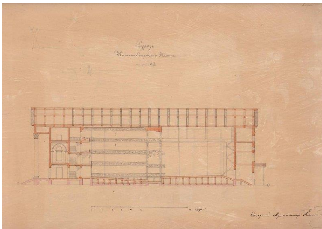
25. Арх. И.И. Климов Иван Иванович. Архитектурный рисунок. Аксонометрический разрез здания Каменноостровского театра (бумага, карандаш, акварель, лак, тушь пером). Последняя треть XIX в. СПбГМТМИ ГИК 3910/6.
