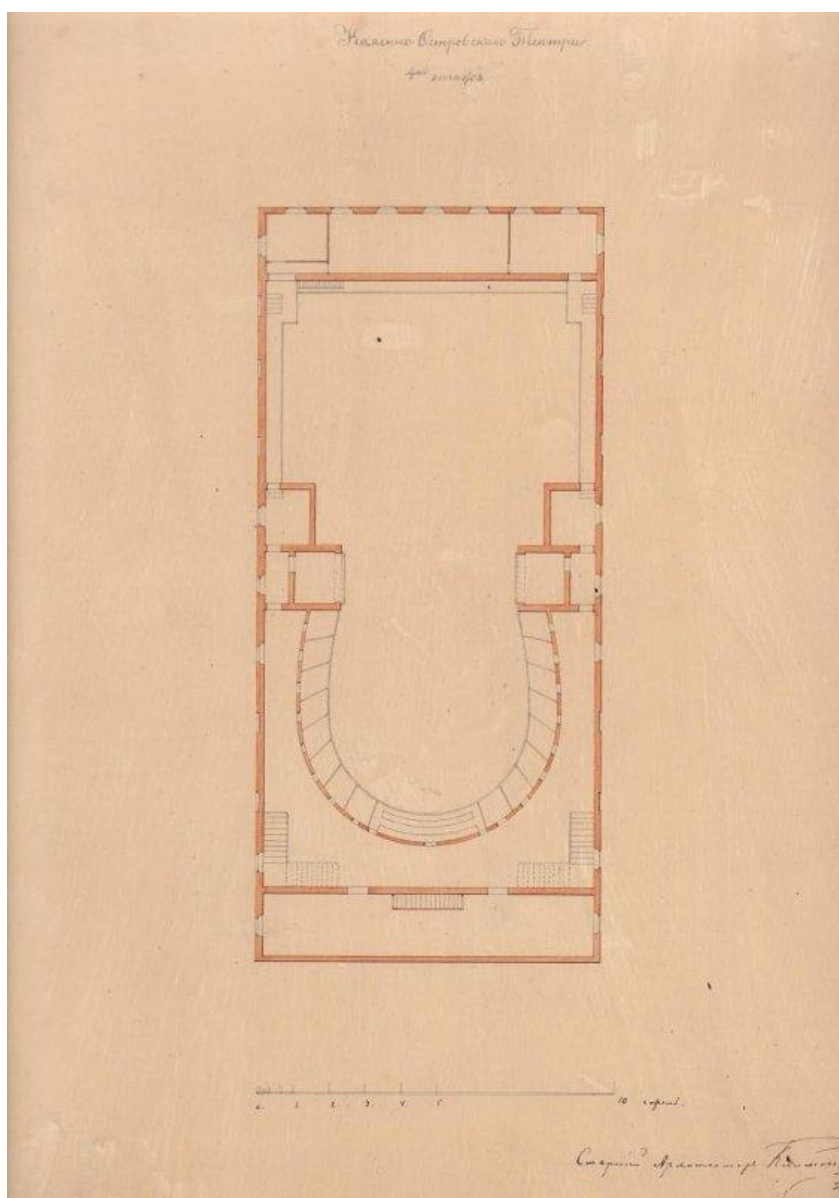
24. Арх. И.И. Климов. План Каменноостровского театра. Четвертый этаж (бумага, тушь пером, акварель). Последняя треть XIX в. СПбГМТМИ ГИК 3910/3.
