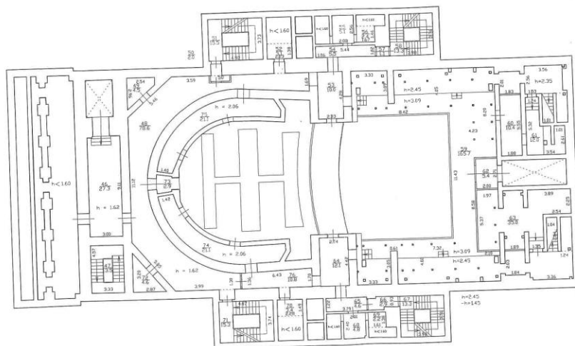
План 1го подземного этажа
