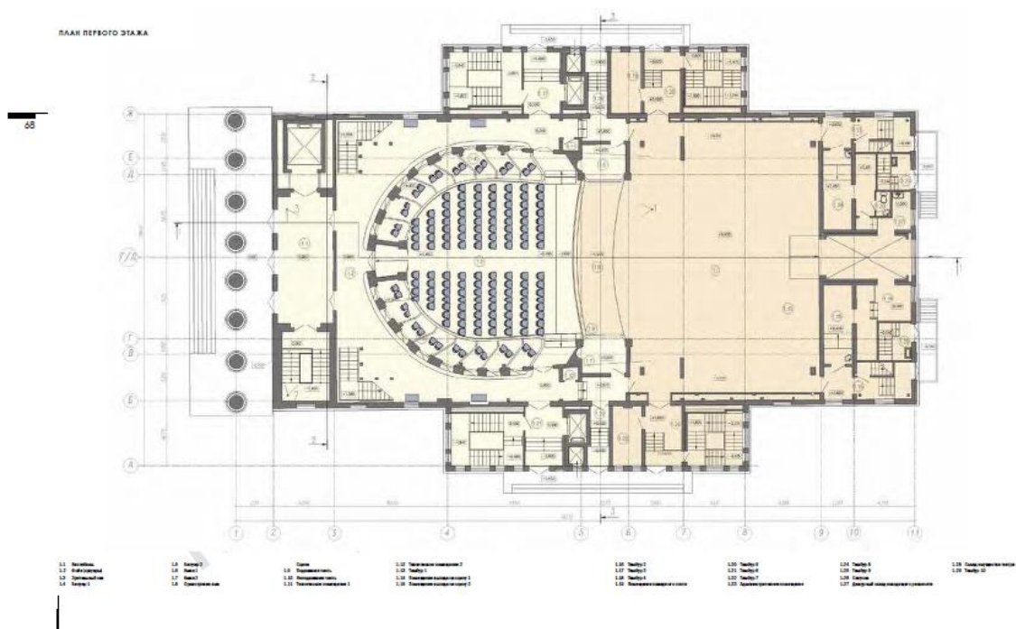
51. Каменноостровский театр. План первого этажа. Проект реставрации приспособления для современного использования. 2007-2011 гг. Опубликовано в: Дементьева В.А., Рахманов В.С., Шашкин А.Г., Бурьгин В.А. Каменноостровский театр. Синтез достижений реставрации и геотехники». (авторы:). СПб., 2014.
