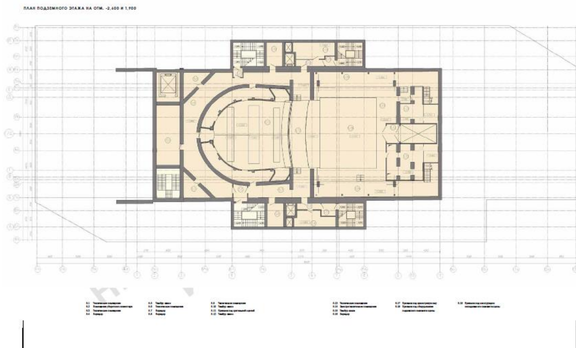
50. Каменноостровский театр. План подземного этажа. Проект реставрации приспособления для современного использования. 2007-2011 гг. Опубликовано в: Дементьева В.А., Рахманов В.С., Шашкин А.Г., Бурьгин В.А. Каменноостровский театр. Синтез достижений реставрации и геотехники». (авторы:). СПб., 2014.
