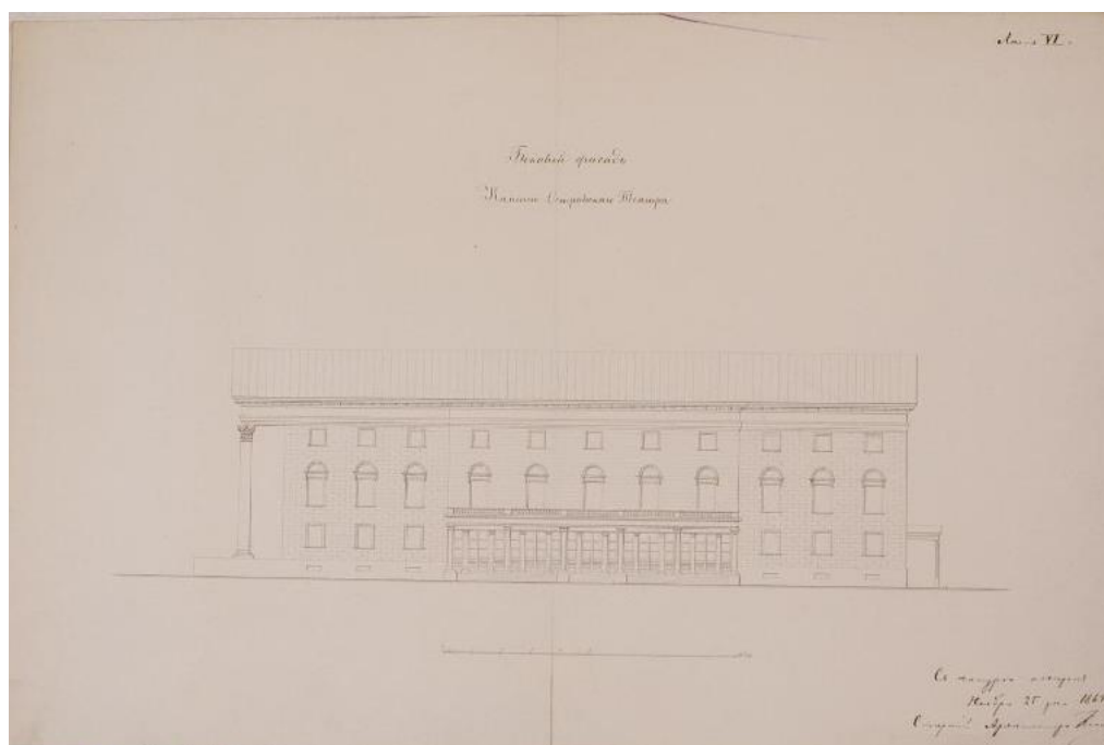
12. Арх. И.И. Климов. Обмер Каменноостровского театра в Санкт-Петербурге (бумага с водяными знаками («i.whatman 1864»), тушь). 1864 г. НИМ РАХ КП-49/26.
