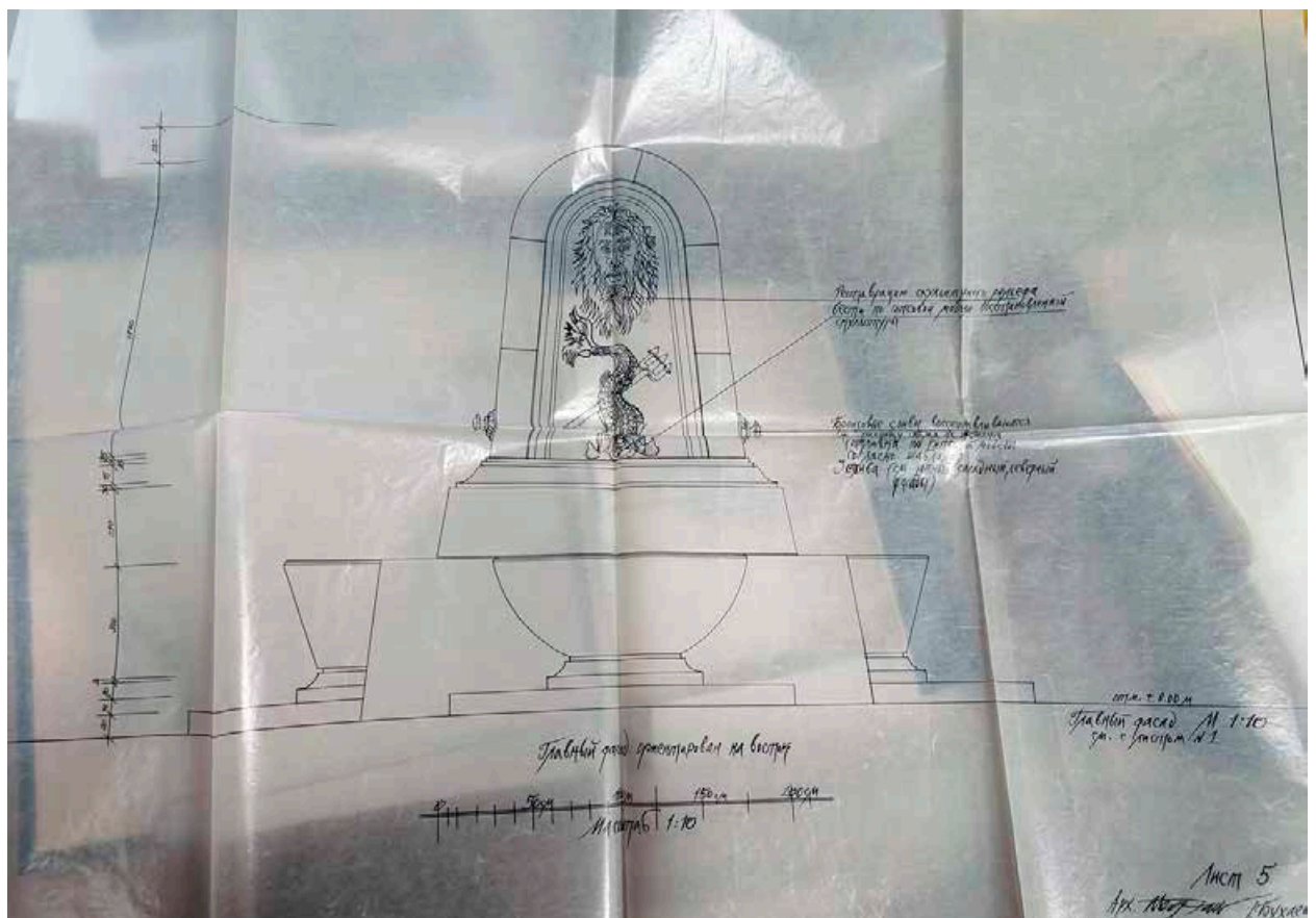
Илл. 16. Фонтан «Нептун». Главный (восточный) фасад. Обмерный чертеж с существующими дефектами. Архитектор В.Б. Бухаев. 1988 г. Архив СПб ГБУК «ГМГС». Д. 33.
