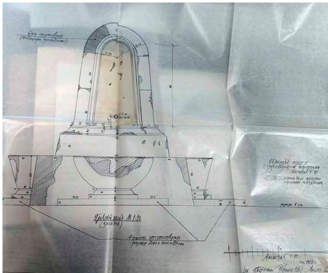
Илл. 17. Фонтан «Нептун». Главный (западный) фасад. Обмерный чертеж с существующими дефектами. Архитектор В.Б. Бухаев. 1988 г. Архив СПб ГБУК «ГМГС». Д. 33.
