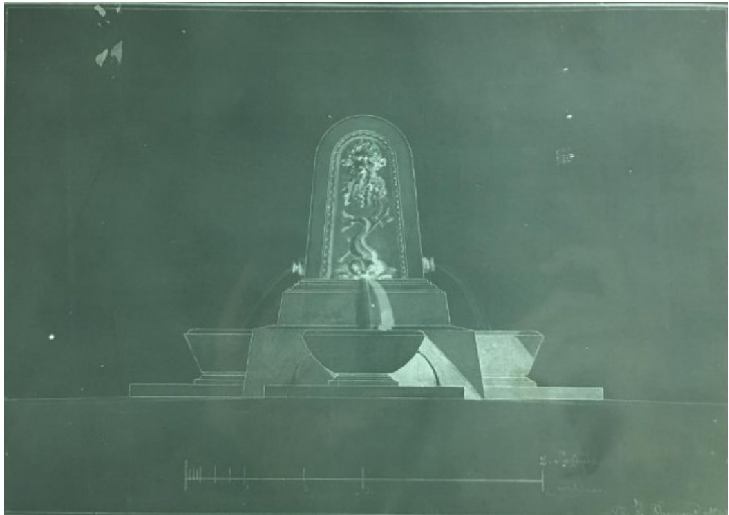
Илл. 1. Фонтан с маской Нептуна на Царскосельской дороге. Чертеж. Архитектор Тома де Томон. 1809 г. ФГБУК «Государственный научно-исследовательский музей архитектуры имени А.В. Щусева». ГНИМА НФ-ОФ-205/297.
