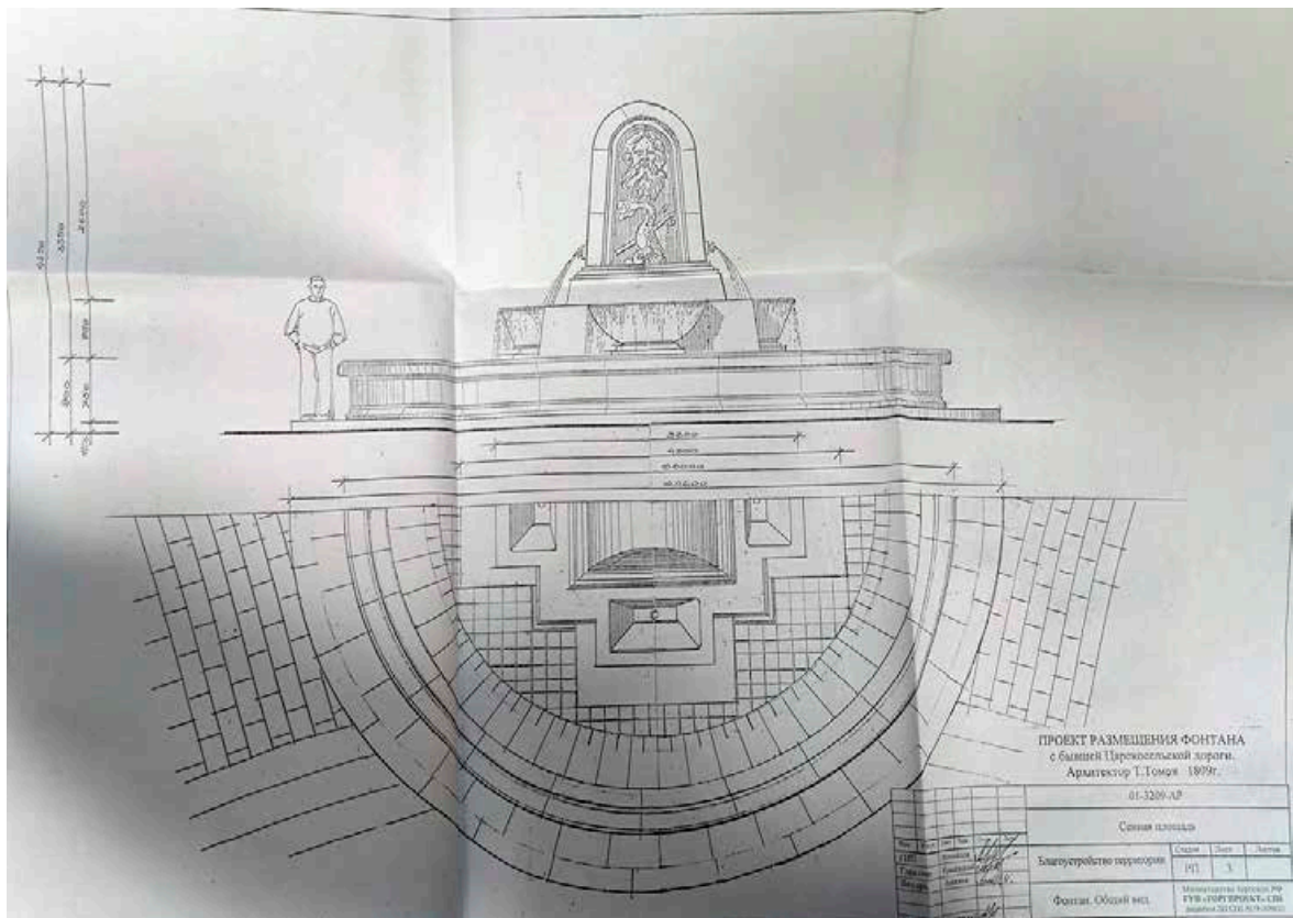
Илл. 20. Проект размещения фонтана на Сенной площади. 2002 г. Архив СПб ГБУК «ГМГС». Д. 33.
