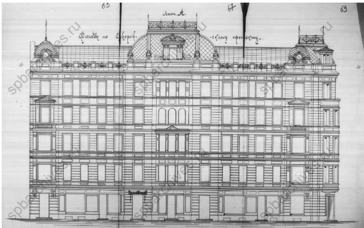
31. ЦГИА СПб. Фонд 515. Опись 4. Дело 5128. Чертежи дома А.Н.Тряничева, П.С.Бочалова, Н.А.Веренчевой, Н.А.Голенищевой по 7-й Рождественской ул.,9,11,13 и Суворовскому пр.,20.
