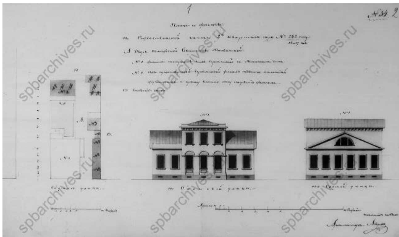
41. ЦГИА СПб. Фонд 513. Опись 102. Дело 9379 Чертежи дома на участке, принадлежавшем А.М.Толвинской, С.Л.Володину, П.С.Бочагову, А.Н.Тряничеву, Н.А.Веренчевой и Н.А.Голенищевой по 7-й
