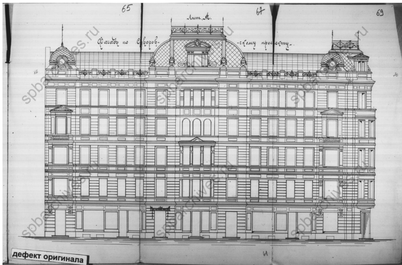
51. ЦГИА СПб. Фонд 515. Опись 4. Дело 5128 Чертежи дома А.Н.Тряничева, П.С.Бочалова, Н.А.Веренчевой, Н.А.Голенищевой по 7-й Рождественской ул., 9, 11, 13 и Суворовскому пр., 20
