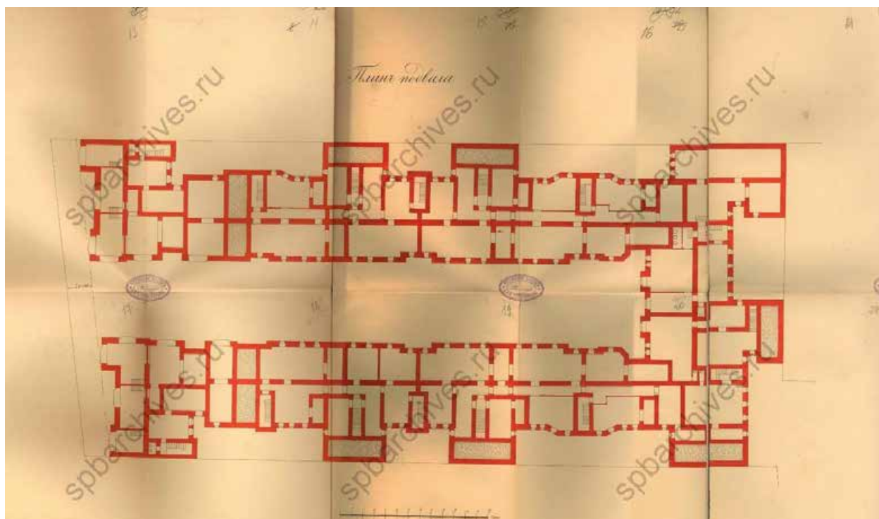
Илл. 13. План подвала. 1911 г. ЦГИА СПб. Ф. 513. Оп. 102. Д. 5300. Л. 13-21, 27.
