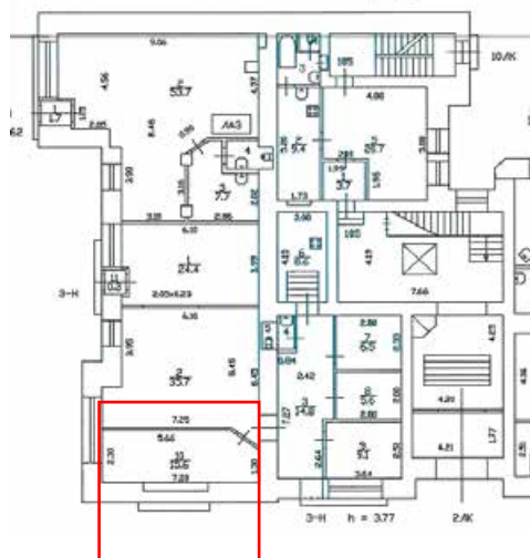
Рис. 4 – План части первого этажа (по состоянию на 14.08.2023 г.). Оконный проем в осях «А/2-3».
