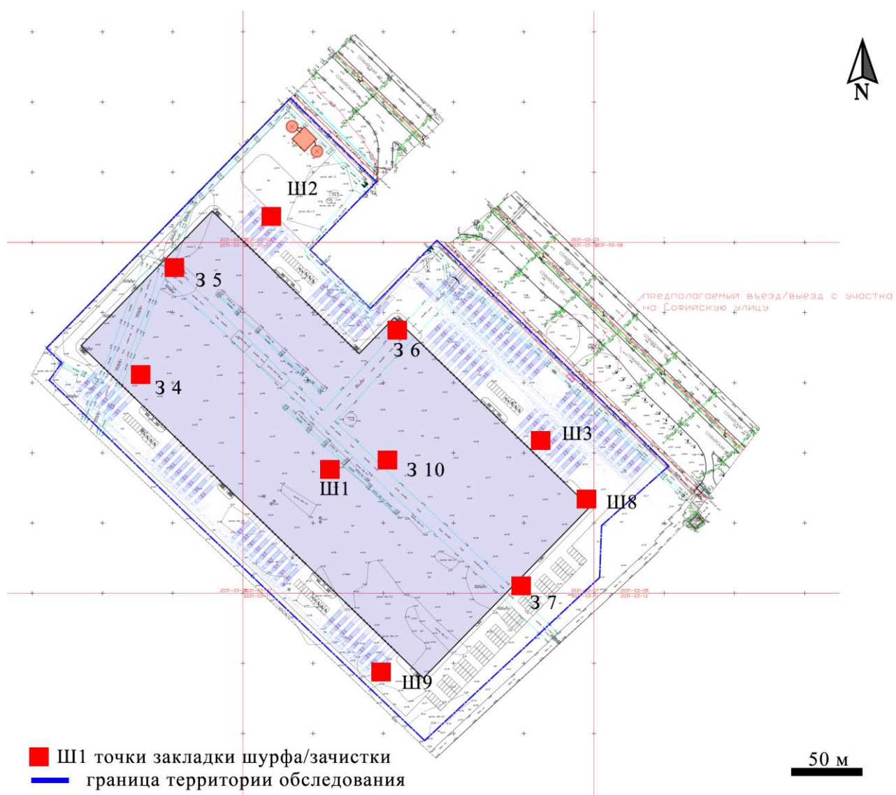
Рис.22. Расположение шурфов и зачисток. Топоъемка предоставлен заказчиком работ.
