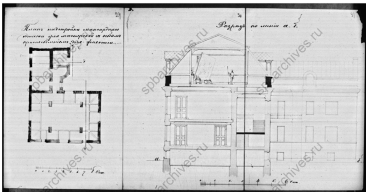
Рис. 11. План 3-го этажа и разрез по линии а. б. 1883 г.
