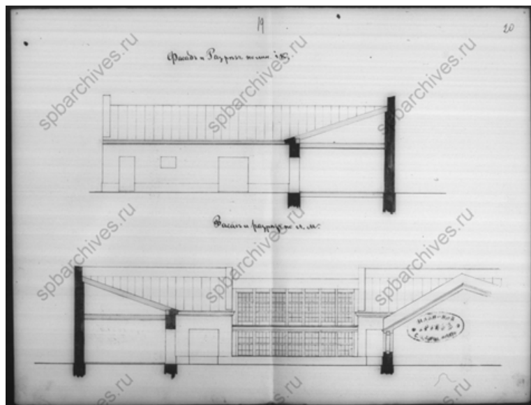
8. Постановление Городской Управы, план двора, принадлежащего Г.Х. Потеста. Фасады, разрезы, поэтажные планы. 11.05.1881 г. ЦГИА СПб. Ф. 513. Оп. 102. Д. 7778. Лл. 15-20.
