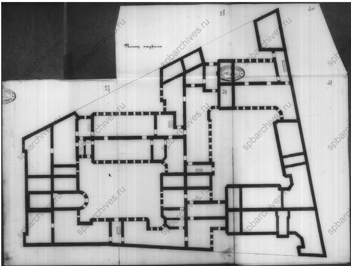
12. План подвала. 1912 г. ЦГИА СПб. Ф. 513. Оп. 102. Д. 7778. ЛЛ. 27-31.
