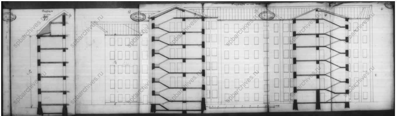
15. Разрезы и дворовые фасады. 1912 г. ЦГИА СПб. Ф. 513. Оп. 102. Д. 7778. ЛЛ. 45-61.
