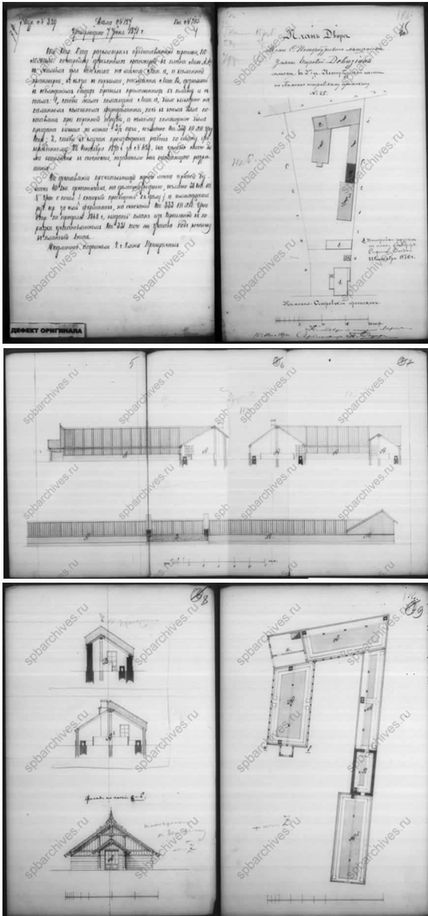
6. Постановление Городской Управы, план двора, принадлежащего У.Е. Дивизион. Фасады, разрезы, поэтажные планы. 07.07.1871 г. ЦГИА СПб. Ф. 513. Оп. 102. Д. 7778. ЛЛ. 4-9.
