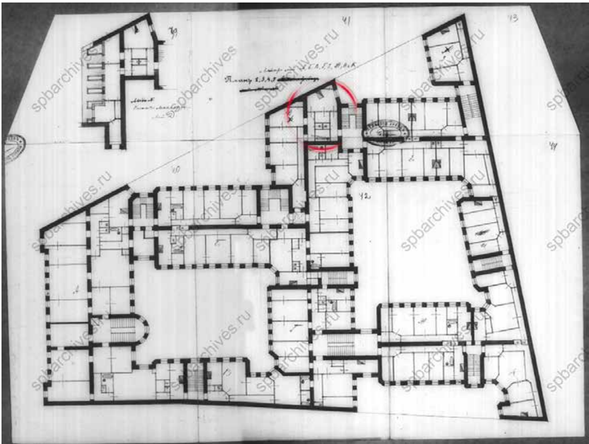
14. План второго-пятого этажей. 1912 г. Примерное расположение современной кв. 66 (2й эт.). ЦГИА СПб. Ф. 513. Оп. 102. Д. 7778. ЛЛ. 39-44.
