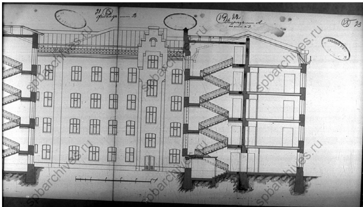
Илл. 15. Разрез лит. А по линии CD. 1904 г. ЦГИА СПб. Ф. 513. Оп. 102. Д. 2512. Л. 21-23.
