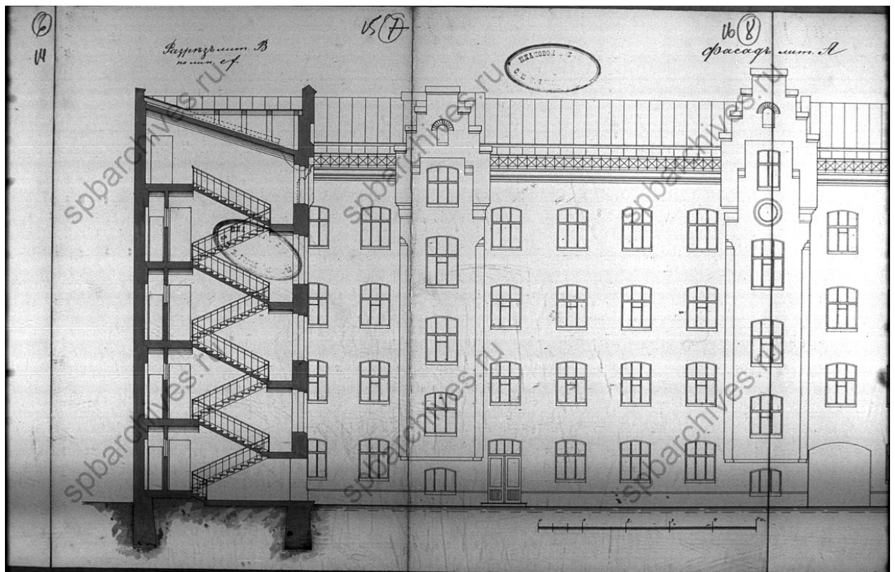
Илл. 13. Фасад лит. А. 1904 г. ЦГИА СПб. Ф. 513. Оп. 102. Д. 2512. Л. 15-16.
