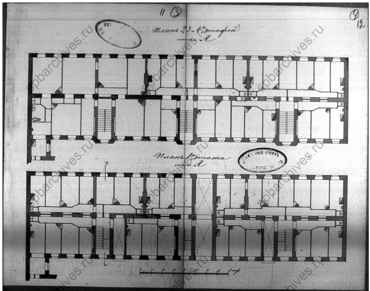
Илл. 12. Планы 1-4 этажей, лит. А. 1904 г. ЦГИА СПб. Ф. 513. Оп. 102. Д. 2512. Л. 11-12.
