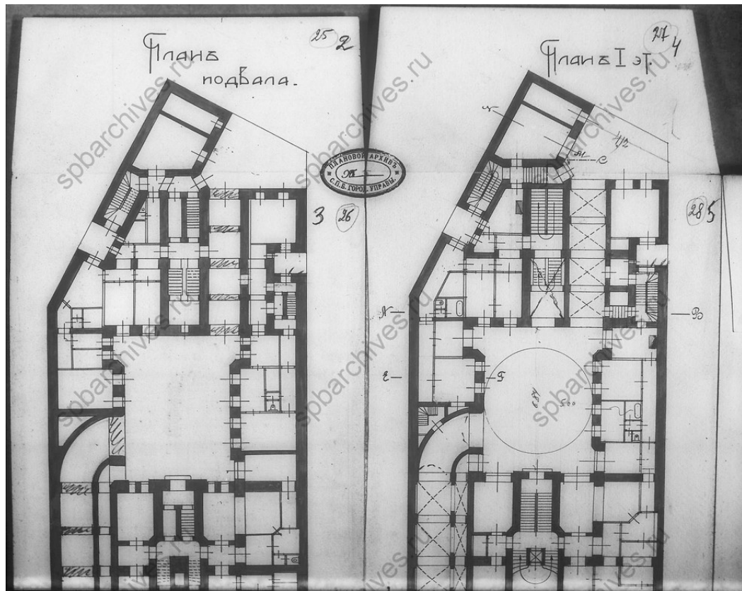
Илл. 13. Планы подвала и 1-го этажа. 1909 г. ЦГИА СПб. Ф. 513. Оп. 102. Д. 9555А. Л. 2-5.
