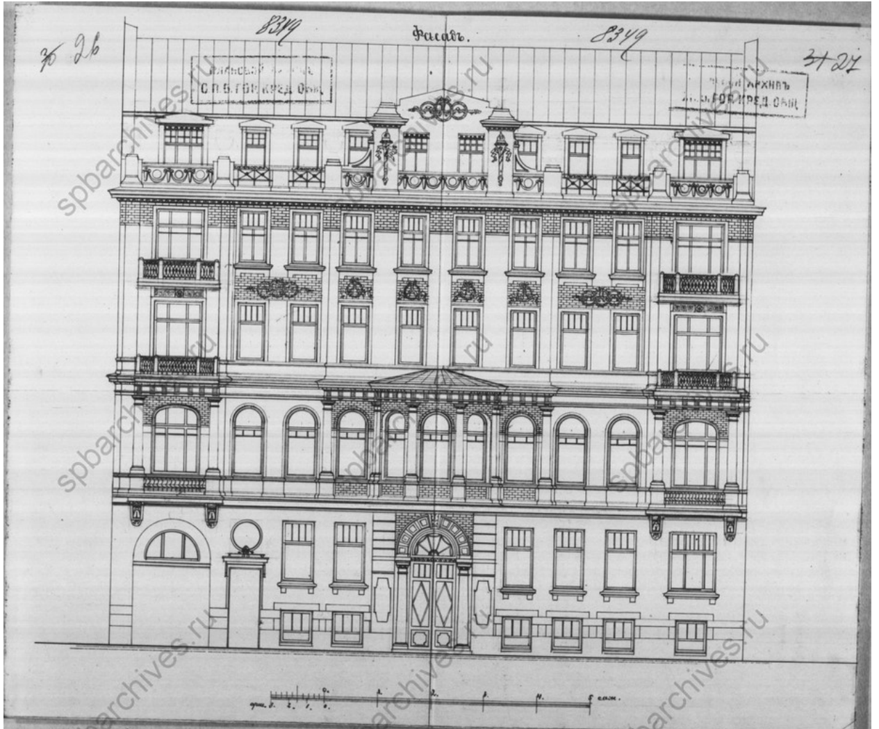
Илл. 39. Фасад. 1910 г. ЦГИА СПб. Ф. 515. Оп. 4. Д. 4978. Л. 26-27.
