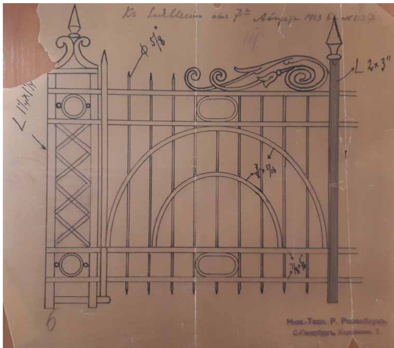
25. Проект решетки вокруг памятника Петру I. 1913 г. ЦГИА СПб., Ф. 1296, Оп. 15, Д. 2. Л. 14
