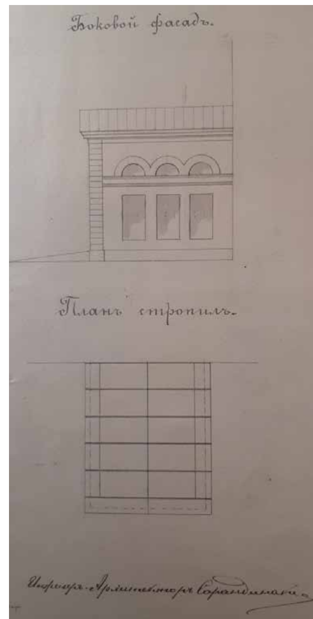
11. Проект пристройки для паровой машины при столярной мастерской. 1889 г. Архитектор В.В. Сарандинаки. ЦГИА СПб., Ф. 1296, Оп. 15, Д. 4. Л. 30-31
