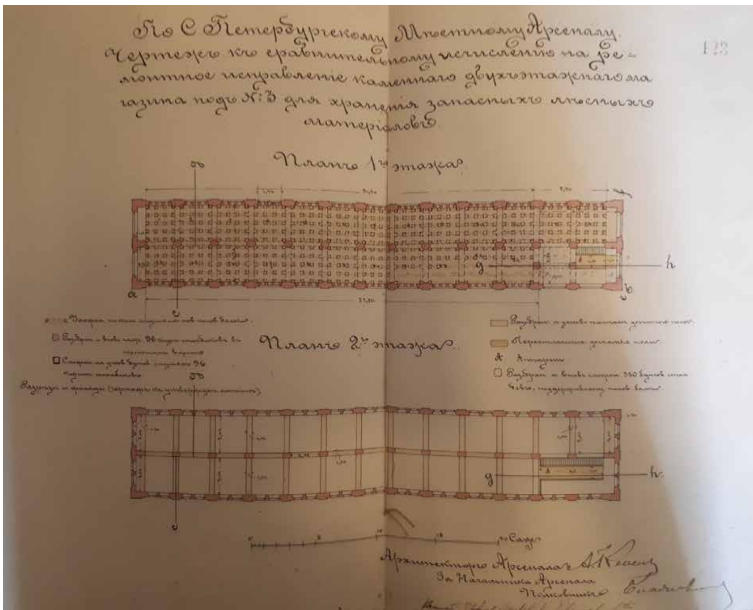
13. Проект исправления каменного магазина № 3. 1901 г. Архитектор А.В. Кенель. ЦГИА СПб., Ф. 1296, Оп. 2, Д. 76. Л. 73
